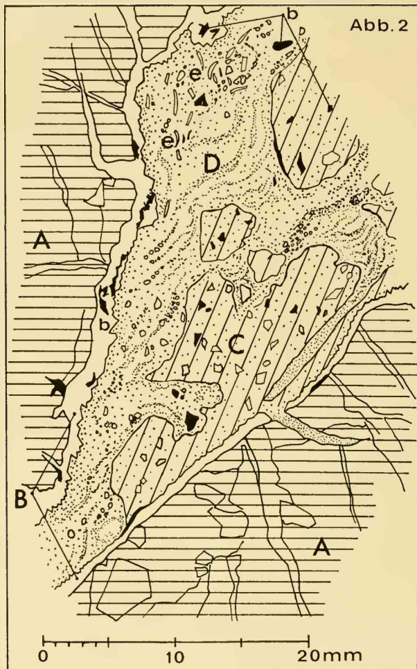
Abb. 2: Karstspalte im Dachsteinkalk mit Kalzitrasen und Gosaaufüllung. A = Dachsteinkalk; B = Kalzitkristalle, welche die Wandung des Hohlraums überziehen; C = stark bauxitisches, peltisches Sediment mit zerbrochenen klaren Kalzitkristallen und dichten Bauxitbröckchen (b); D = eingeschwemmtes Gosaaus sediment mit aufgearbeiteten Brocken aus C, reichlich Schalenschutt (e = Reste von Erymnaria ) und Bauxitbröckchen (b). Schliff G 1022 a/68.
