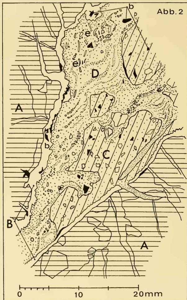
Abb. 2: Karstspalte im Dachsteinkalk mit Kalzitrasen und Gosaaufüllung. A = Dachsteinkalk; B = Kalzitkristalle, welche die Wandung des Hohlräume überziehen; C = stark bauxitisches, pelitisches Sediment mit zerbrochenen klaren Kalzitkristallen und dichten Bauxitbröckchen (b); D = eingeschwemmtes Gosaaus sediment mit aufgearbeiteten Brocken aus C, reichlich Schalenschutt (e = Reste von Erymnaria ) und Bauxitbröckchen (b). Schliff G 1022 a/68.
