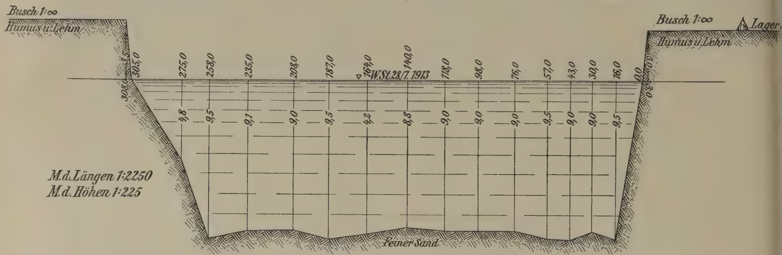
Querprofil des Djah, 1 km oberhalb seiner Einmündung in den Ssanga. V = 0,581 m/sec Oberflächengeschwindigkeit. Q = 1568 cbm/sec.
