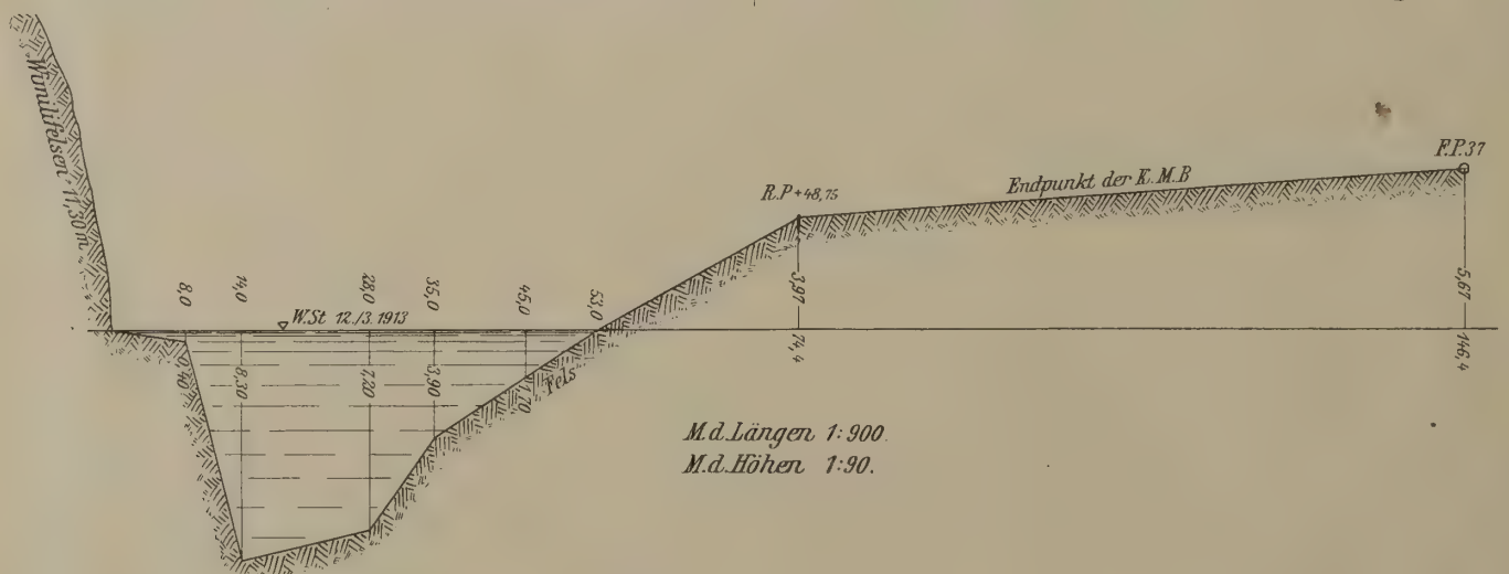
Querprofil des Njong beim Wimilifelsen, 500 m unterhalb des Dorfes Mbalmajo, Kilometer 0. Projektierte Übergangsstelle der Kameruner Mittellandbahn nach dem Süden.
