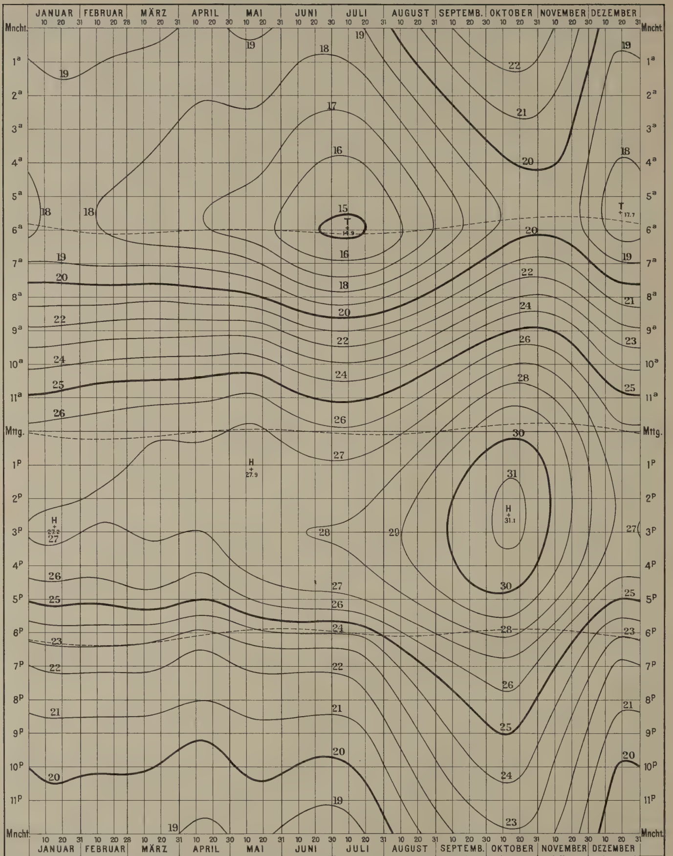
--- Kurven des scheinbaren Aufgangs, der Kulmination und des scheinbaren Untergangs der Sonne nach mittlerer Ortszeit.
