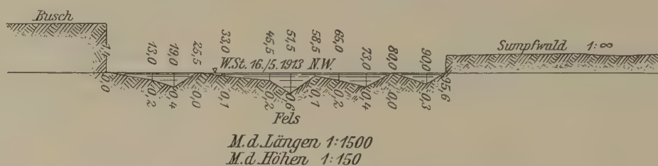
Querprofil des Dume bei den Schnellen von Molambi.
