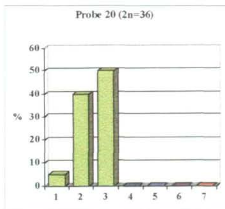
Abb. 4: Cardenolidzusammensetzung der diploiden (Probe 19), tetraploiden (Probe 20), pentaploiden (Proben 21-24) und hexaploiden (Proben 25-28) Mustern von Ornithogalum sp. aus "Südtirol". Strophallosid (1), Convallatoxin und Convallosid (2), unbekannte Strophanthidinglykoside (3), Rhodexin A und Rhodexosid (4), Peripallosid (5), Lokundjosid (6), "rote Cardenolide"(7).
