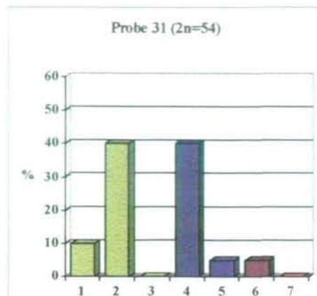
Abb. 6: Cardenolidzusammensetzung der hexaploiden Muster aus dem Handel (Probe 31) und aus Wien (Probe 32). Strophallosid (1), Convallatoxin und Convallosid (2), unbekannte Strophanthidinglykoside(3), Rhodexin A und Rhodexosid (4), Peripallosid (5), Lokundjosid (6), "rote Cardenolide"(7).
