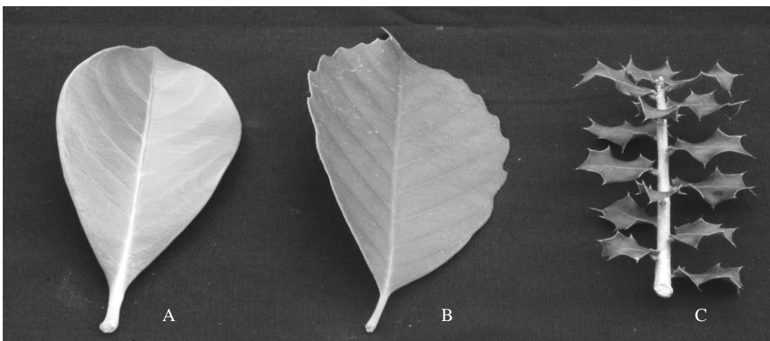
Fig 29: Lithocarpus edulis (A) und Quercus glauca (B) (vgl. Tab. 1) repräsentieren den ursprünglichen, laurophyllen, Quercus coccifera (C) den abgeleiteten, xeromorphen Blattpyus in der Eichen-Verwandtschaft.
