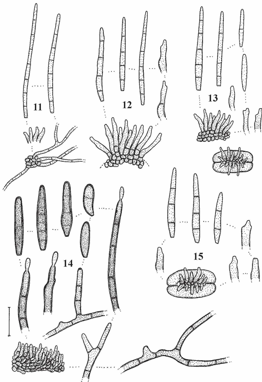
Figs 11-15: Conidiophore fascicles, conidiophores, conidia, 11 – Pseudocercospora paludicola , 12 – P. pareirae , 13 – P. platensis , 14 – Exosporium puccinioides , 15 – Pseudocercospora sapiicola , scale = 20 µm, U. Braun del.
