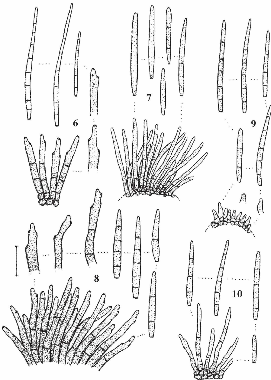
Figs 6-10: Conidiophore fascicles, conidiophores, conidia. 6 – Cercospora furfurella , 7 – Pseudocercospora guaranítica , 8 – Passalora leprosa , 9 – Pseudocercospora mate , 10 – P. megalopotamica , scale = 20 \mu m, U. Braun del.
