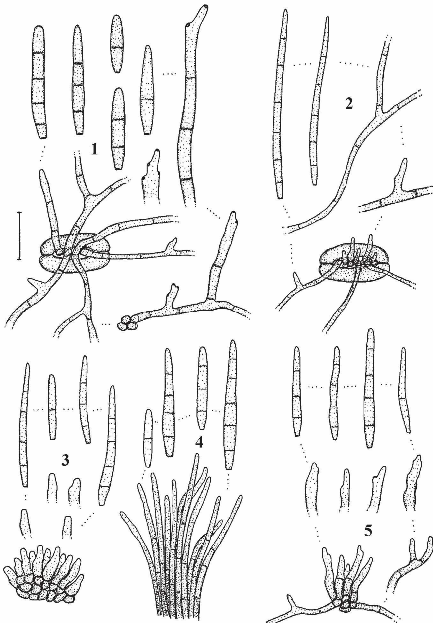
Figs 1-5: Conidiophore fascicles, conidiophores, conidia, 1 – Passalora balansae , 2 – Pseudocercospora bomplandiana , 3 – P. brachypoda , 4 – P. cucurbitina , 5 – P. fumosa , scale = 20 \mu m, U. Braun del.
