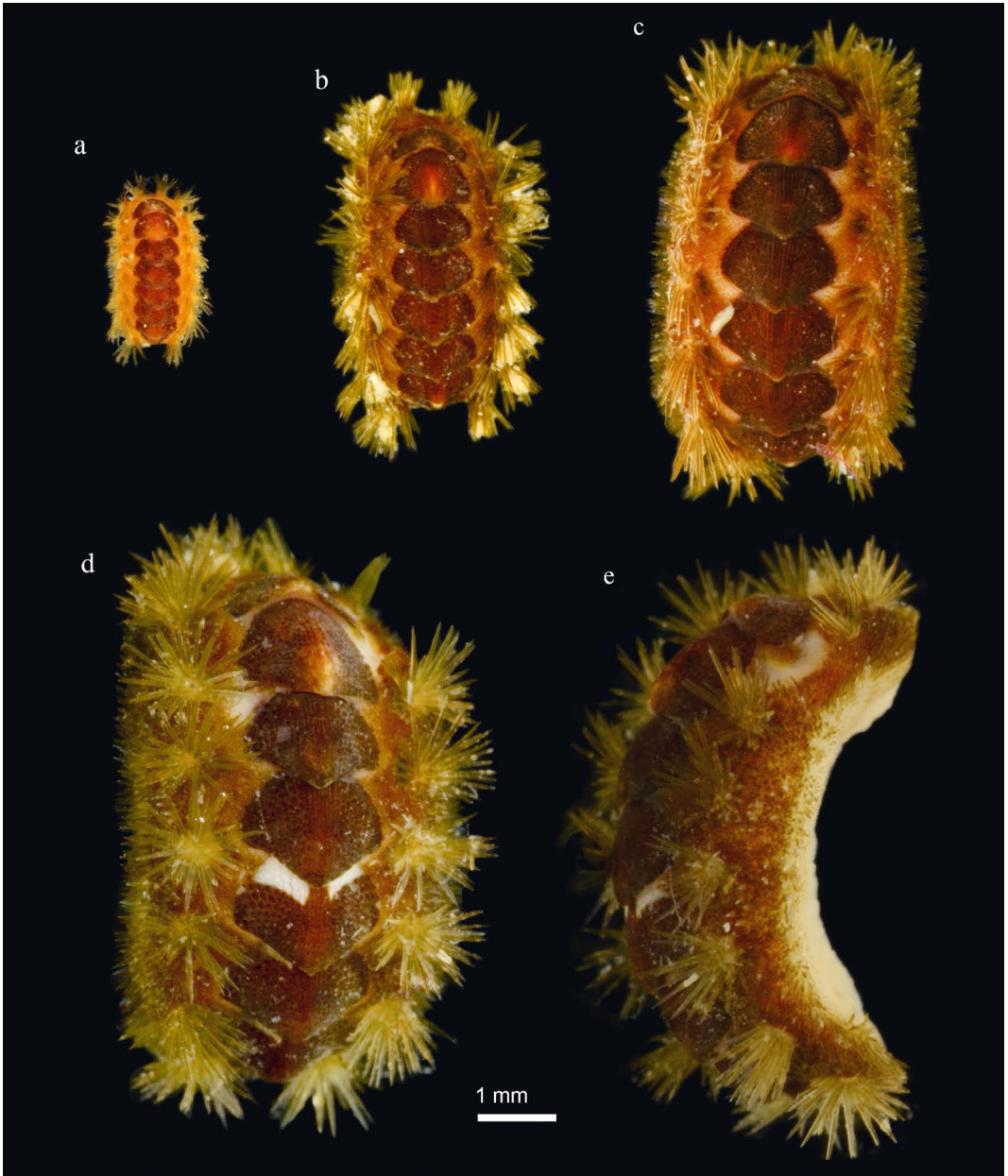
Fig. 4. Different growth stages of Acanthochitona pilosa spec. nov. a. Length 3 mm (ZSM Mol 20034395). b. Length 5 mm (ZSM Mol 1996589). c. Length 7 mm (ZSM Mol 1996589). d,e. Length 9 mm (ZSM Mol 1996589).
