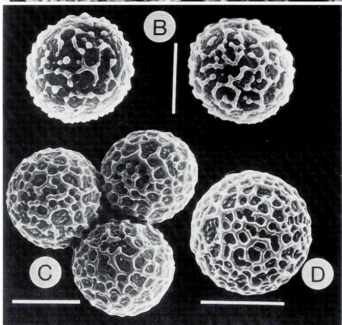
Plate 7. – SEM pictures of Lamprospora ascospores. – A–D. L. minuta . A: Spitsbergen 35 (O); B: Spitsbergen 33 (O); C: D 154/84 (O); D: D203/83 (O). – Bar = 10 \mu m.
