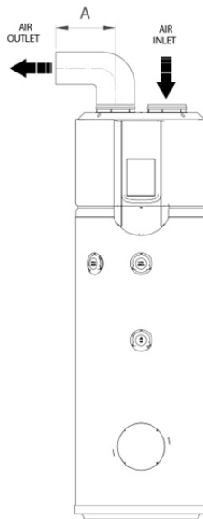
D: Kanalisierte Absonderung ( A \leq 5m )
