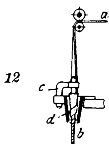
12 Trichter (m) mit eingesetztem Kegeldorn funnel with an inserted conical core воронка (жр) со вставленным коническим стержнем entonnoir (m) comprenant un noyau conique imbuto (m) con anima conica embudo (m) con núcleo interior cónico / embut (m) amb nucli interior cònic
