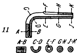
11 Rundungstrichter (m) rounding funnel воронка (жр) для свертывания entonnoir (m) à arrondir imbuto (m) per arrotondare embudo (m) deredondear / embut (m) d'arrodonar
