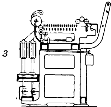
Vorspinnmaschine (f) für Seide silk fly frame, silk roving frame банкаброш (мр) для шелка banc (m) à broches à soie, banc à ailettes à soie banco (m) a fusi per seta mechera (f) / metxera (f) / de seda
