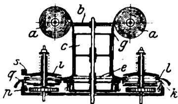
Listersche zwei- köpfige Seiden- kämmaschine (f)
