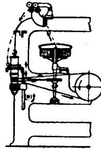
Doppeldrahtspinnmaschine (f) double twist spinning machine
