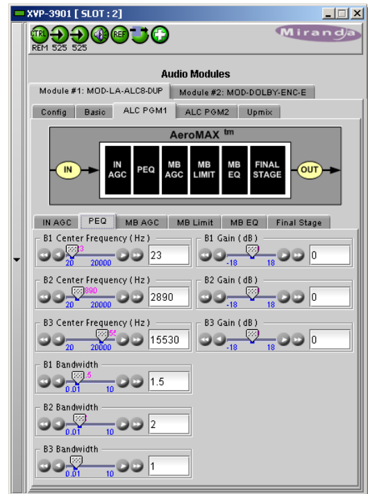
Figure 6.13 ALC - PEQ Parameters
