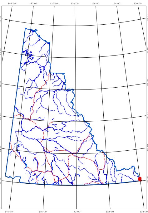
Alisma triviale
