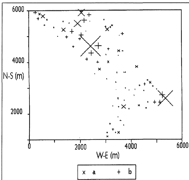
Slika 2: Grafični prikaz napake ocene debeline naplavine a: podcenjena vrednost, b: precenjena vrednost. Fig. 2: Diagrammatic presentation of the error in the alluvium thickness estimate a: underestimated value, b: overestimated value.
