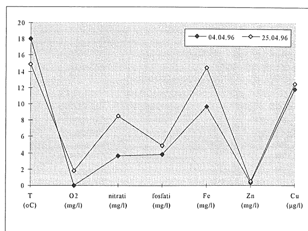
Slika 3: Temperatura (T), vsebnost raztopljenega kisika (O 2 ), nitratov, fosfatov, železa (Fe), cinka (Zn) in bakra (Cu) v sveži izcedni vodi (4.4.1996) in v izcedni vodi, ki je dalj časa satala v kotanji na robu smetišča (25.4.1996).
