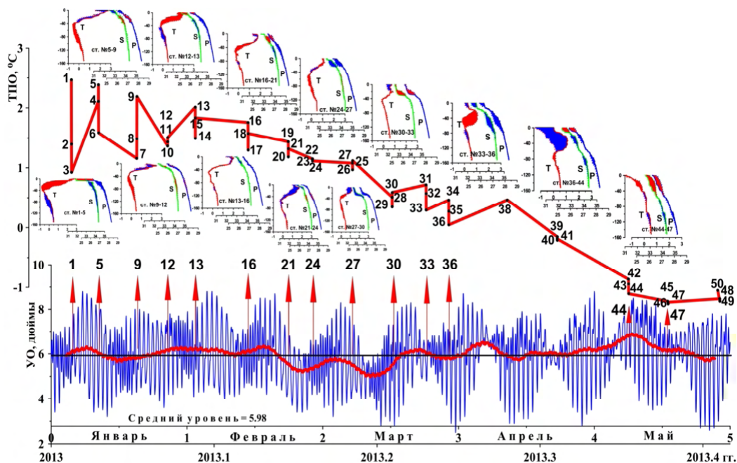
Рис. 4. Временной ход температуры воды на поверхности (ТПО, °С) по всей совокупности гидрологических станций, выполненных в январе-мае 2013 г., и уровень океана (УО, дюймы) у станции Академик Вернадский. Стрелками показано положение станций на оси времени, числа над стрелками – номера станций. Жирная кривая – УО, сглаженный скользящим средним по семи суткам. На врезках – вертикальные профили температуры (Т), солёности (S) и плотности (P) для станций, выполненных в проливе Пенола (эти станции выделены прямоугольником на рис. 2). Профили совмещены попарно для двух последовательных станций, номера которых приведены на рис. 2). Профили совмещены попарно для двух последовательных станций, номера которых приведены на графиках. Левая ось – глубина (м), нижние оси – Т (°С), S (‰), P (усл. ед.).
