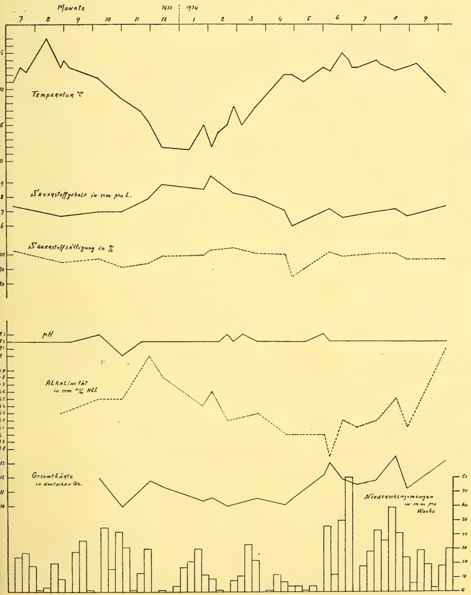
Fig. 7e. Mittellauf des Röserenbaches bei Quelle 13.
