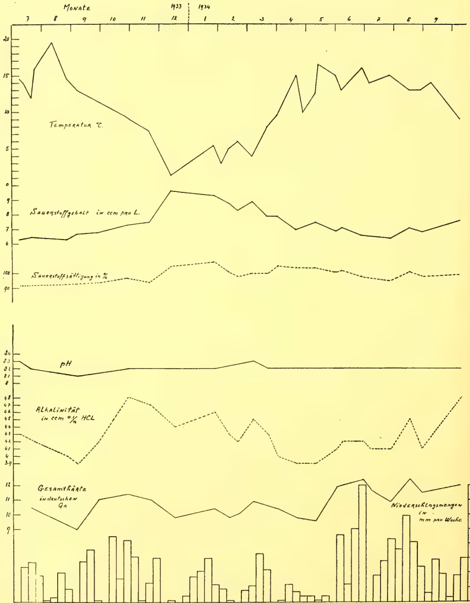
Fig. 7f. Unterlauf des Röserenbaches zwischen Quelle 16 und 17.
