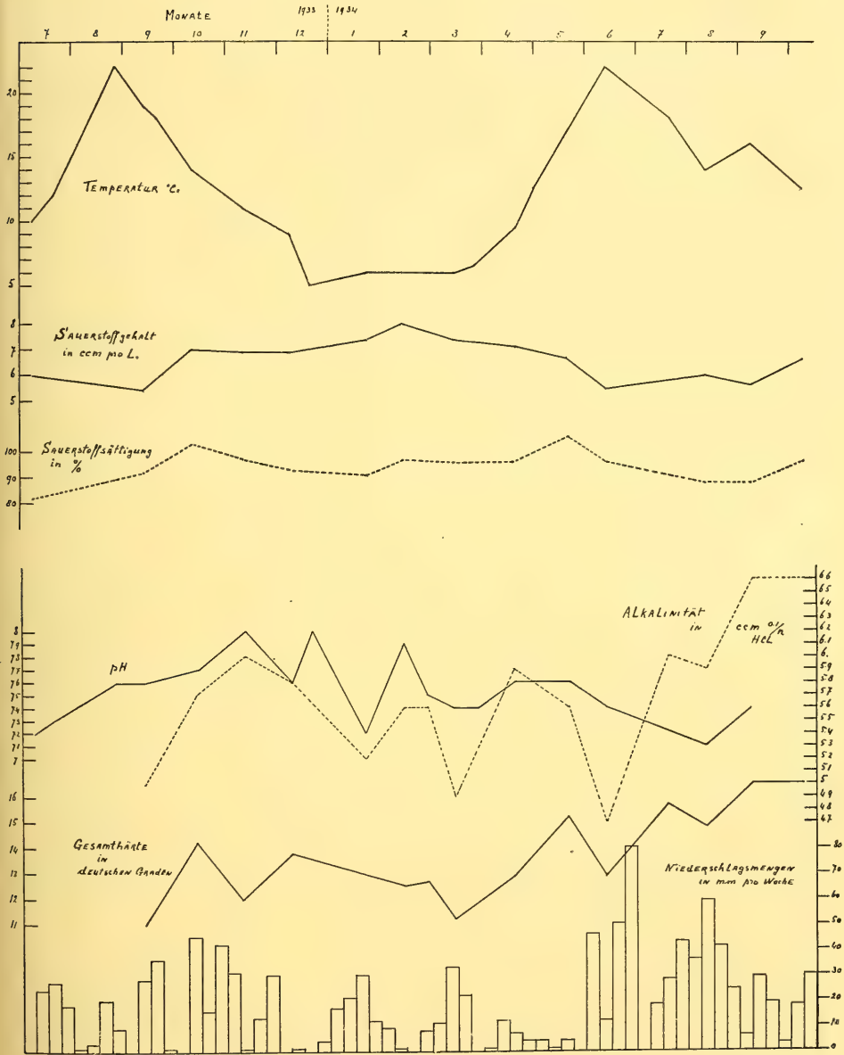
Fig. 7a. Quelle 1, wasser arme Limmokrene (Tugmatt) der Rauracienkalke.
