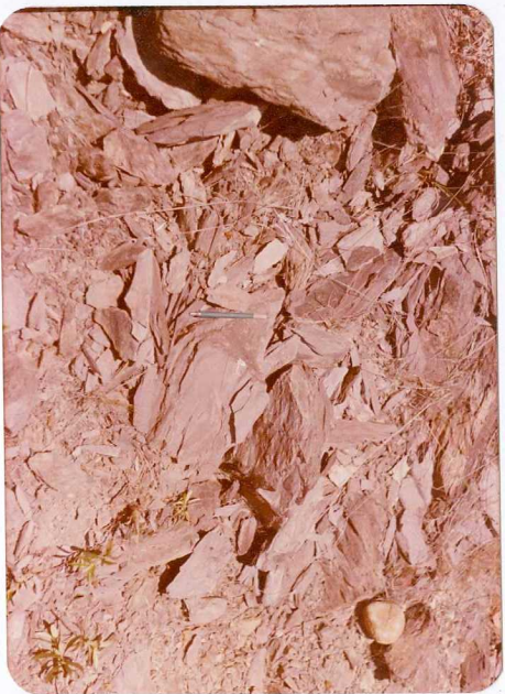
10-38-AD-CO-237: Pizarras moradas correspondientes al nivel guía que pasa junto al Embalse de agua - agria de Riotinto.
