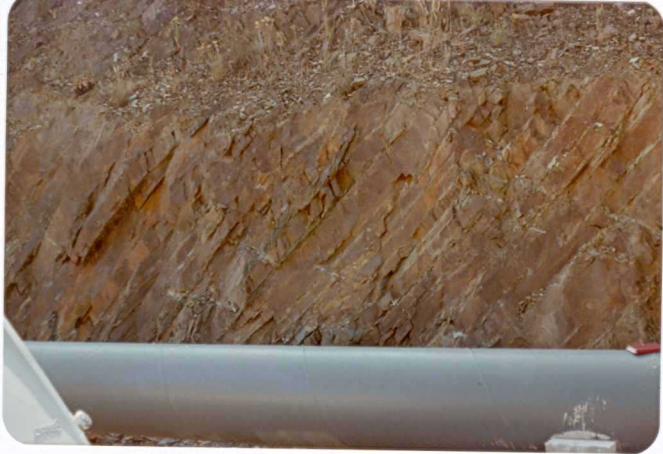
10-38-AD-CO-239: Alternancia de pizarras y grauwacas del Vi seense. Ctra. Dehesa-Campofrío.
