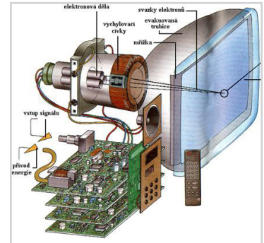
Televizní CRT obrazovka
