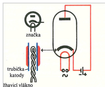
Nepřímo žhavená elektronka Zapojení a schematická značka.
