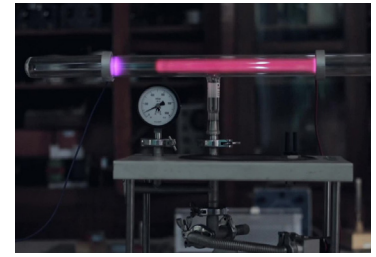
Výbojová trubice spojená s vývěvou
