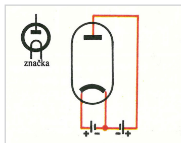
Přímo žhavená elektronka Zapojení a schematická značka.
