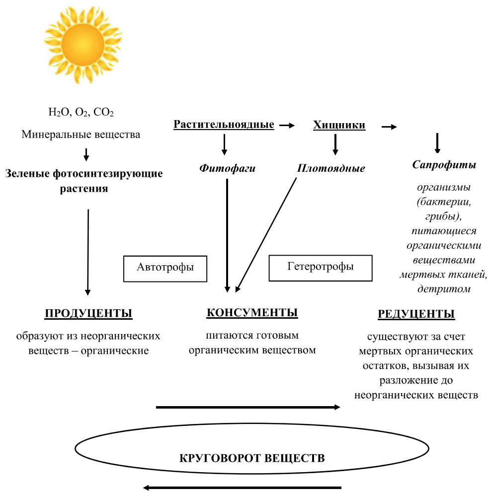
Рисунок 6 – Структура биоценоза
