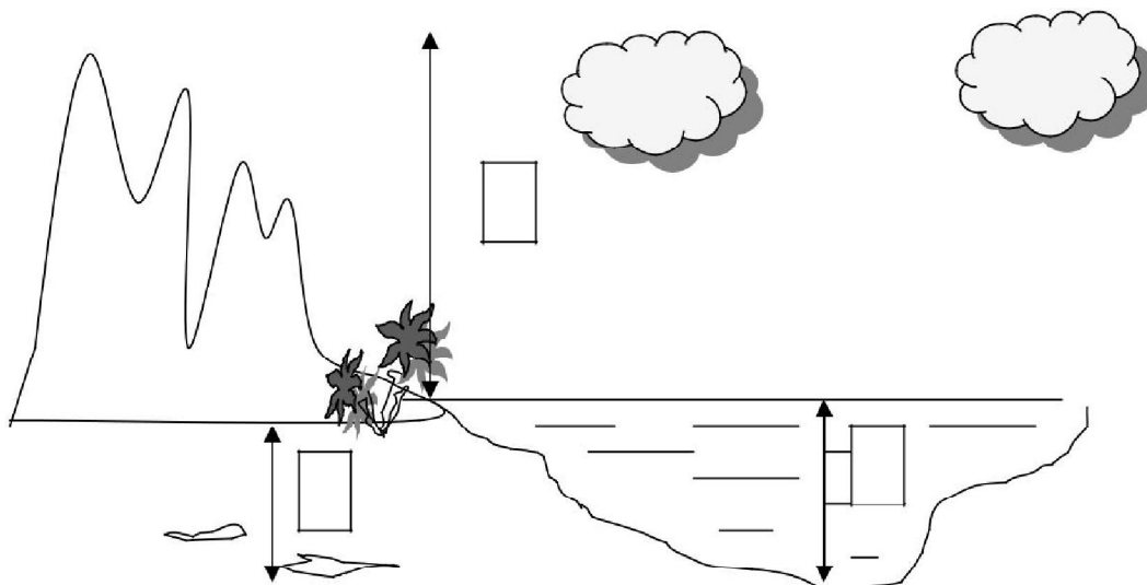
Рисунок 1 – Границы биосферы
