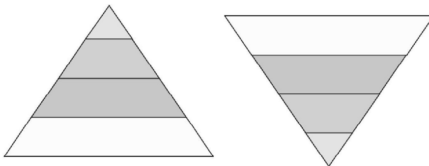
Рисунок 3 – Экологические пирамиды
