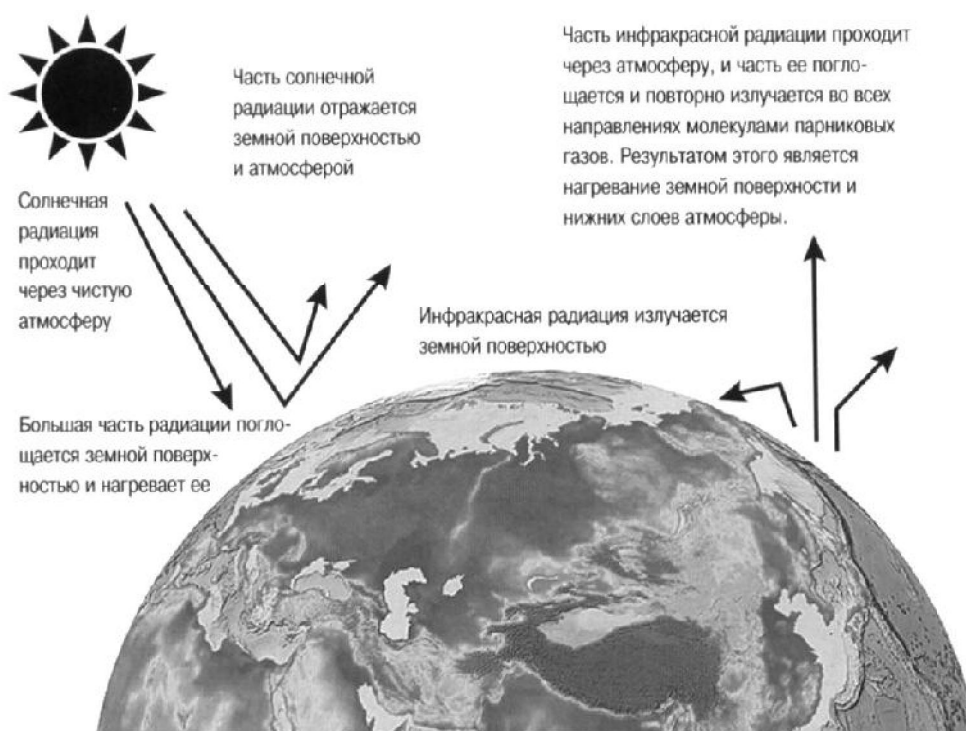
Рисунок 10 – Схема парникового эффекта (по материалам брошюры ЮНЕП «Изменение планеты»)
