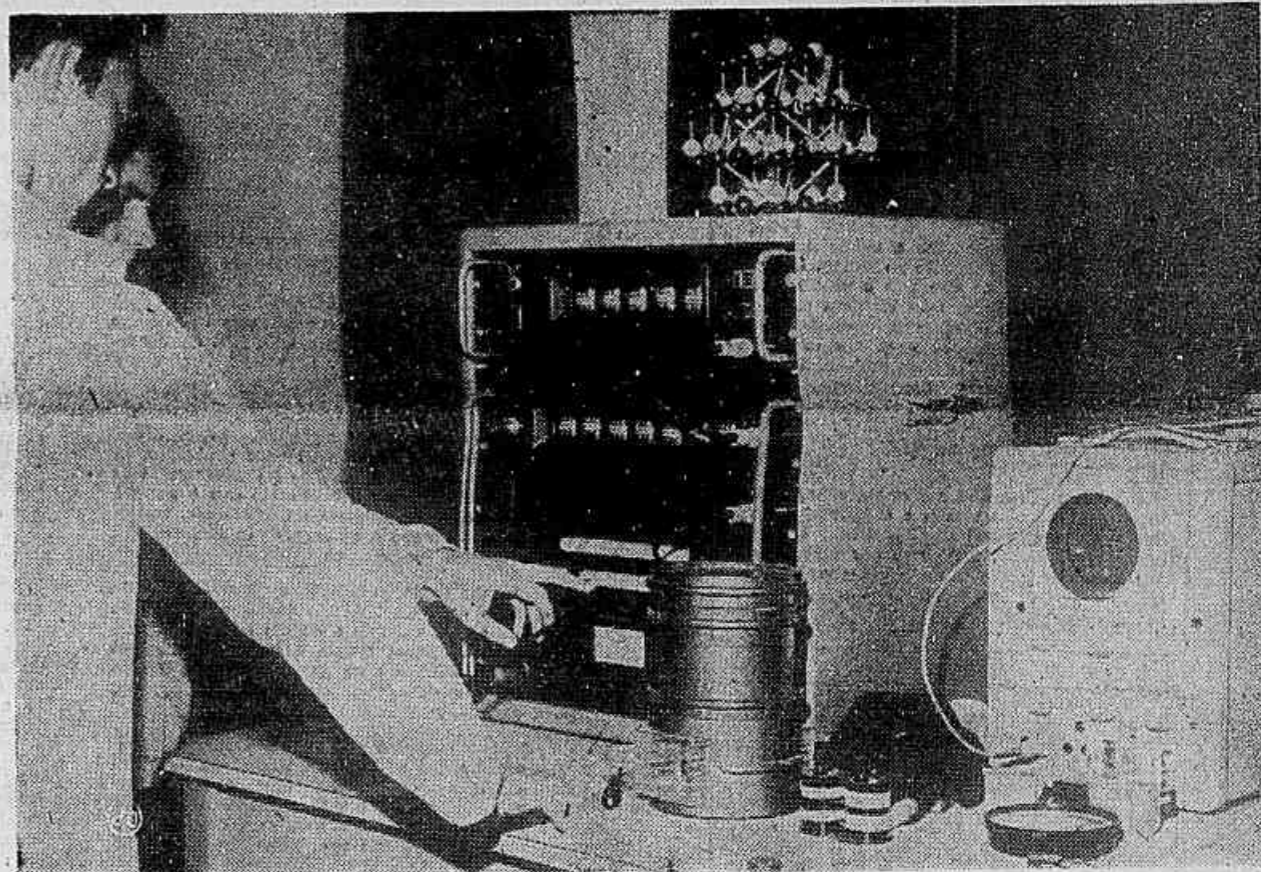
Físicos da UFP estudam as correntes atmosféricas, mas es-tão abalissados a dizer que a garoa nuclear está presente.
