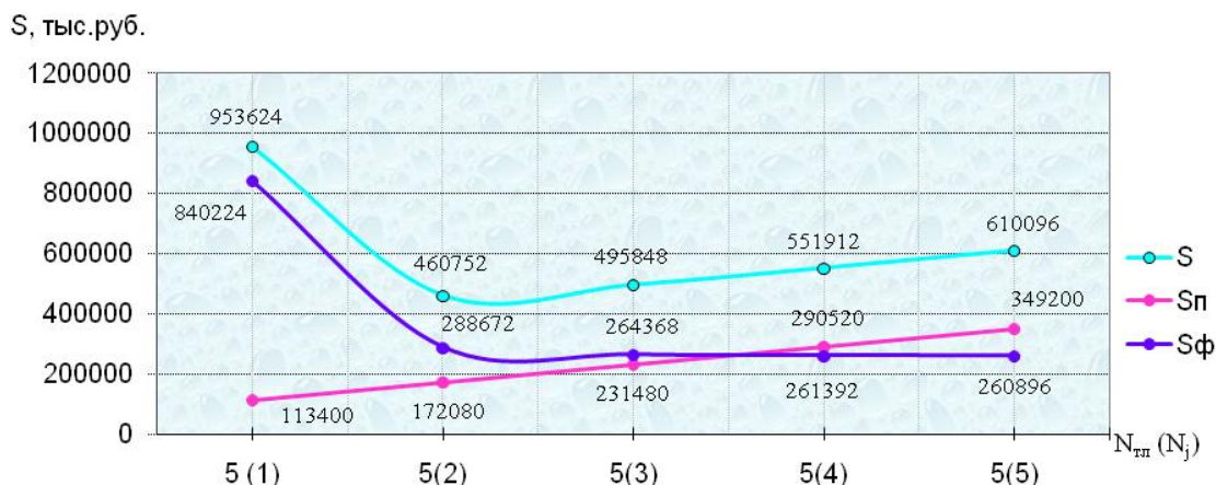
Рис. 1. График зависимости приведенных затрат от N_{ТЛ} и N_J .
