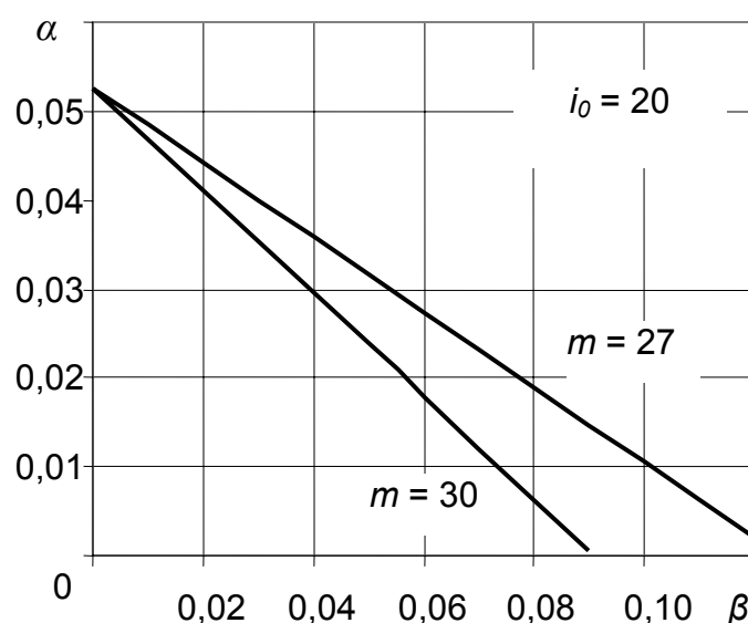
Рис. 1. Диаграмма изменения среднего возраста судов в составе флота ( \tau = 0 )
