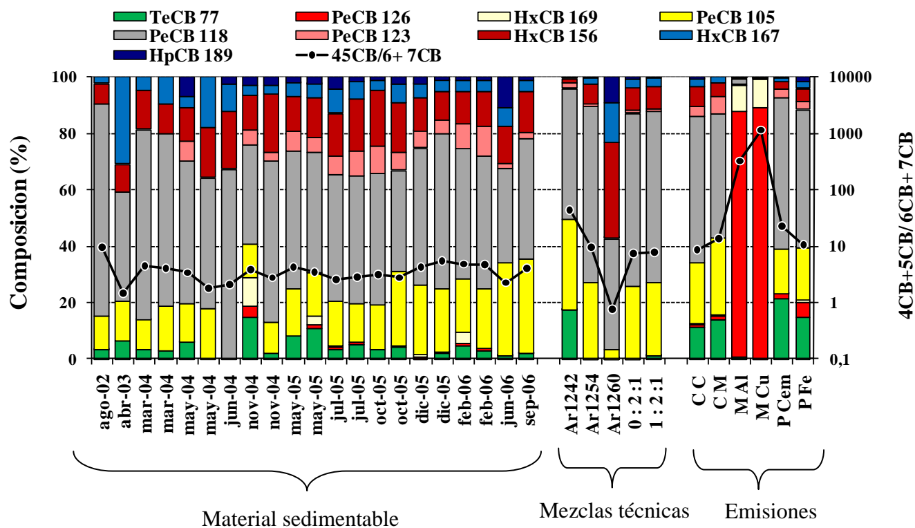
Figura 16. Composición de diPCB y relación 4+5CB / 6+7CB en el material en sedimentación en BZ, formulaciones técnicas Aroclor (Ar) incluyendo mezclas entre 1242, 1254 y 1260 (0:2:1 y 1:2:1, respectivamente), emisiones de combustión de carbón (CC) y madera (CM), plantas metalúrgicas de aluminio (MAI) y cobre (MCu), producción de cemento (PCem) y hierro (PFe).
