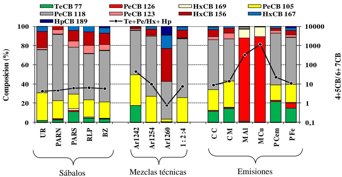
Figura 18. Composición de dlPCB y relación 4CB_{Te}+5CB / 6CB+7CB en sábalos de de los ríos Uruguay (UR), Paraná norte (PARN), Paraná Sur (PARS), Río de la Plata (RLP), y Berazategui (BZ) y mezclas técnicas Aroclor (Ar), emisiones provenientes de combustión de carbón (CC) y madera (CM), plantas metalúrgicas de aluminio (MAI) y cobre (MCu), producción de cemento (PCem) y hierro (P Fe).
