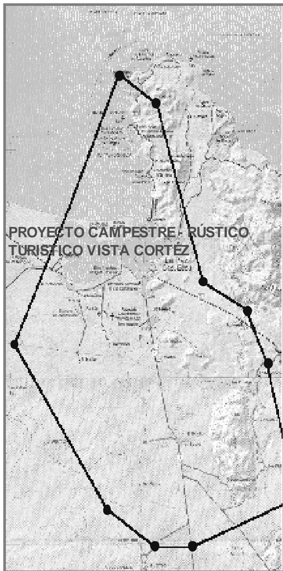
Figura 22 .Cuenca de La Paz y subcuencas donde se localiza Proyecto Campestre rústico "Vista Cortéz"
