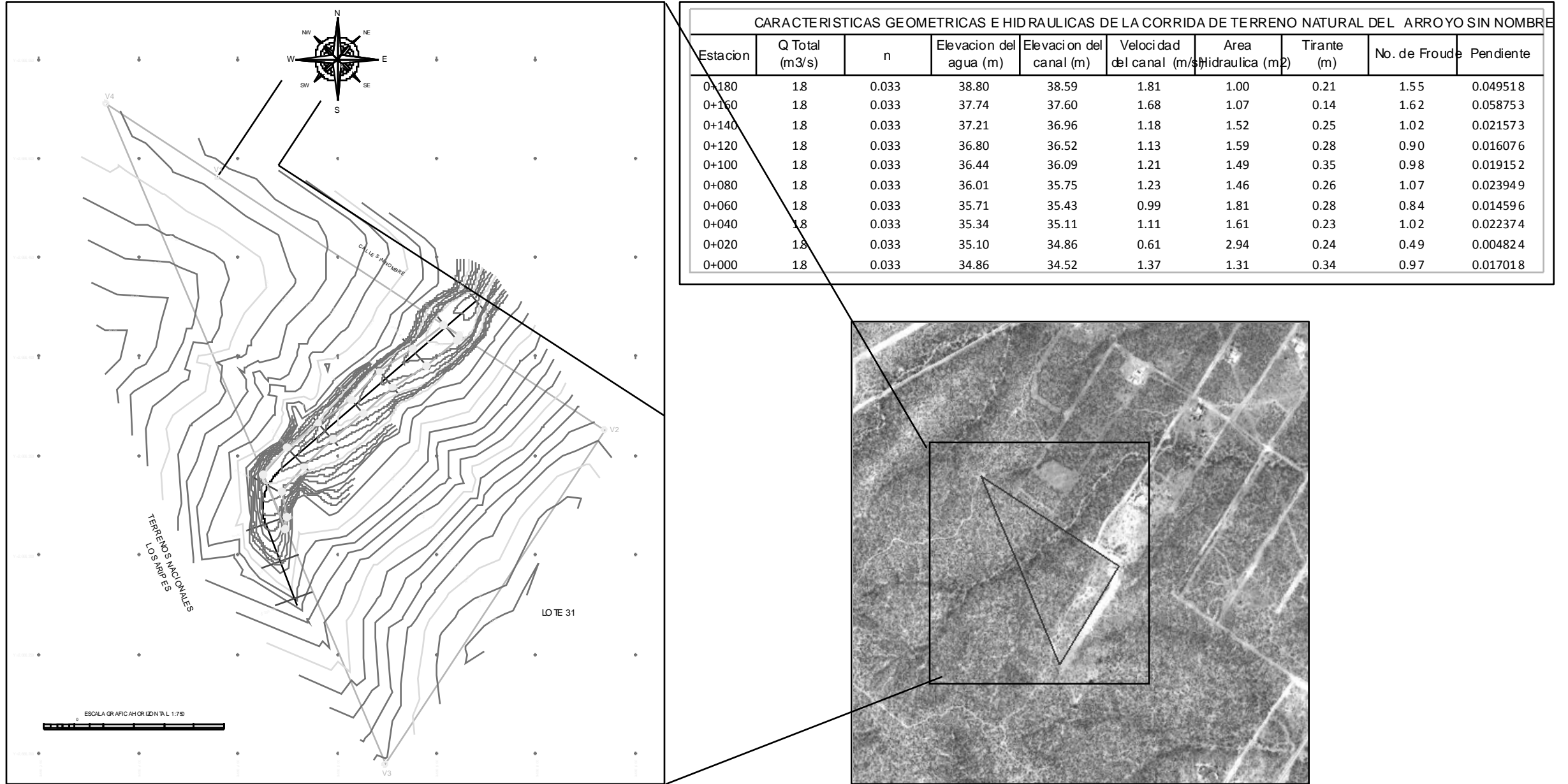
Figura 23. Configuración topográfica y características geométricas e hidráulicas del arroyo s/n, proyecto Campestre Rústico Vista Cortéz
