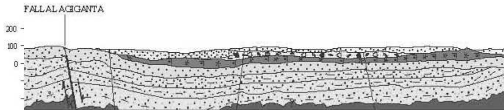
Figura 21. Sección Geológica del Valle de La Paz, incluyendo los límites tectónicos de la cuenca. Falla de La Paz al este y falla de la Giganta al oeste. Como se observa en la sección el proyecto Vista Cortéz se localiza en el centro - oeste de la cuenca de La Paz, en lomeríos bajos conformados por material detrítico de conglomerado polimictico del Pleistoceno.
