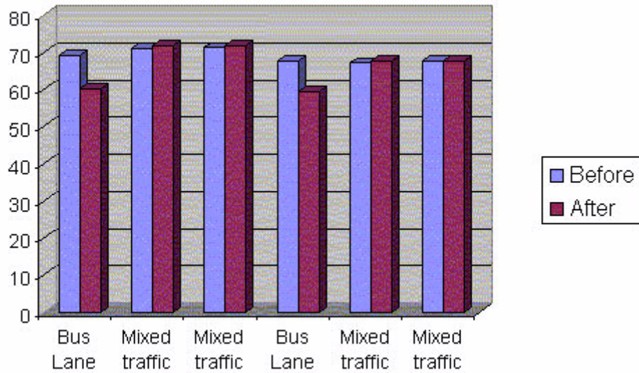
Εικ. 19: Επίπεδα θορύβου, ανά λωρίδα, για την Εγνατία πριν και μετά την εισαγωγή των λεωφορειολωρίδων για το ύψος των 4m
