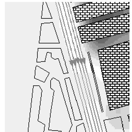
Εικ. 29: Επίδραση της απόστασης στη στάθμη L_{10(18h)}
