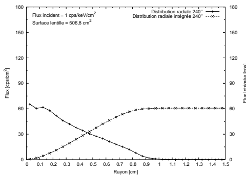
(e) Dépointage : 4 arcminutes
