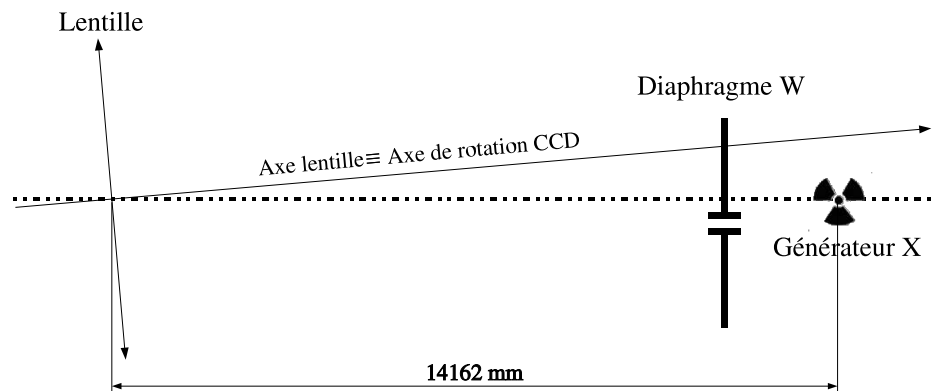
(a) Etape 1 : Avant alignements
