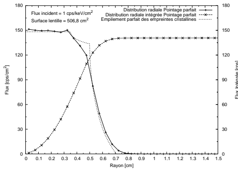
(a) Pointage parfait
