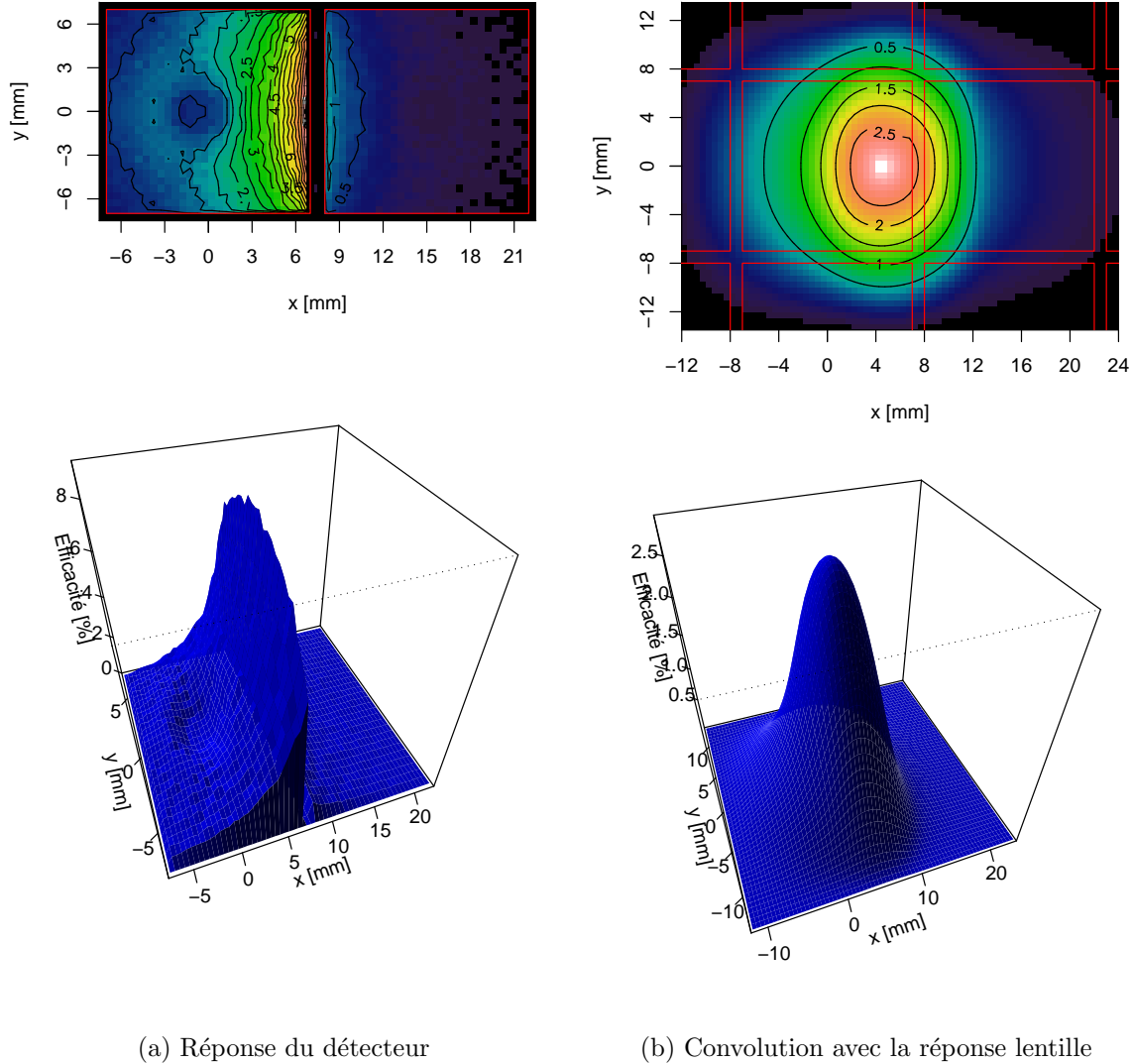
FIG. 3.14: Simulation de l'efficacité de détection pour les évènements doubles (énergie reconstituée entre 160 et 170 keV).
