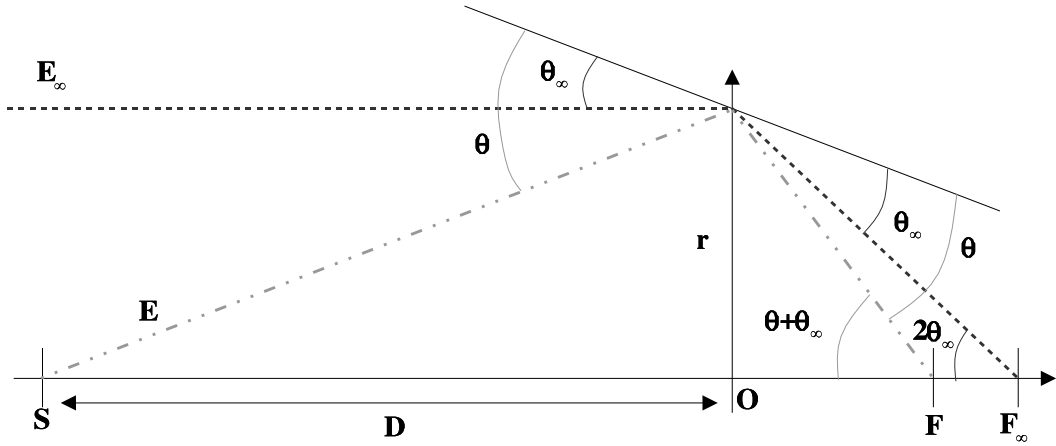
FIG. 2.17: Schéma de principe d'une lentille \gamma
