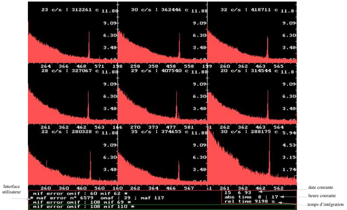
(a) Les neufs détecteurs simultanément
