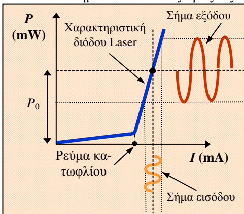
Σχ. 4.4.8. Χαρακτηριστική οπτικής ισχύος εκπομπής – ρεύματος πόλωσης διόδου Laser. Η διαμόρφωση του ρεύματος οδήγησης της Laser από το σήμα πληροφορίας, μετατρέπεται από το γραμμικό τμήμα της καμπύλης σε αντίστοιχες διακυμάνσεις της οπτικής ισχύος εξόδου.
