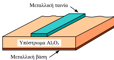
Σχ. 4.3.1. Βασική δομή μικροταινίας.
