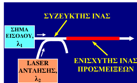
Σχ. 4.6.2. Ενισχυτής ίνας προσμείξεων. Ο συζευκτής ίνας εισάγει τα δύο μήκη κύματος στον πυρήνα της ίνας προσμείξεων.
