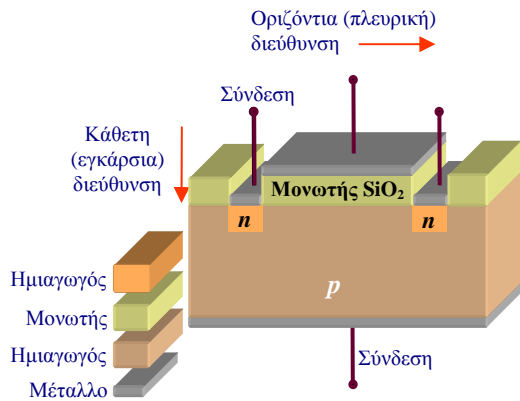
Σχ. 4.2.7. Σχηματικό διάγραμμα τρανζίστορ ολοκληρωμένου κυκλώματος.
