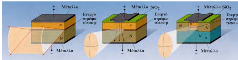
Σχ. 4.4.6. Διάφοροι τύποι ημιαγωγικών laser.
