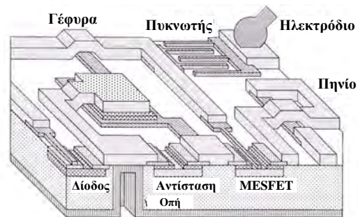
Σχ. 4.3.2. Τριδιάστατο σχηματικό διάγραμμα MMIC.
