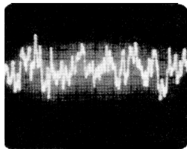
Σχ. 3.1.2. Ο ηλεκτρονικός θόρυβος στη άκρη ενός χάλκινου ζεύγους όπως φαίνεται στον παλμογράφο.
