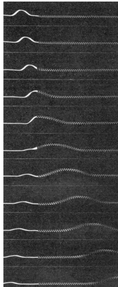
Σχήμα 1.4.3. Ένας παλμός που μεταδίδεται στο ελατήριο και συναντά το σταθερό άκρο, ανακλάται. Αν στο σταθερό άκρο συνδεθεί ένα άλλο ελατήριο με διαφορετικά χαρακτηριστικά (βαρύτερο ή σκληρότερο π.χ.), τότε στη ζεύξη, δηλαδή στο σύνορο μεταξύ των δύο ελατηρίων, ο παλμός χωρίζεται. Στο σχήμα φαίνονται δύο συνδεδεμένα ελατήρια, ένα βαρύ ελατήριο στα αριστερά και ένα ελαφρότερο στα δεξιά. Ο παλμός ταξιδεύει στο αριστερό ελατήριο με κατεύθυνση στα δεξιά. Στη ζεύξη ο παλμός και διέρχεται και ανακλάται μερικώς.
