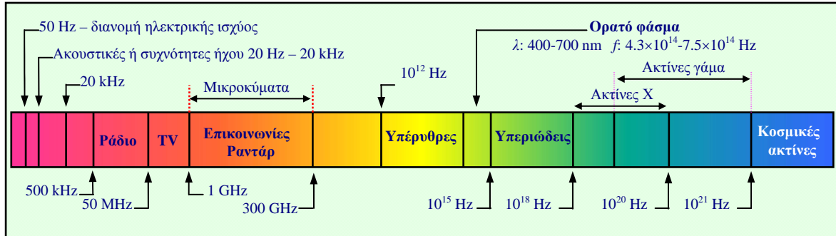
Σχ. 3.3.3. Οι κυριότερες περιοχές του ηλεκτρομαγνητικού φάσματος και η χρήση της κάθε περιοχής.
