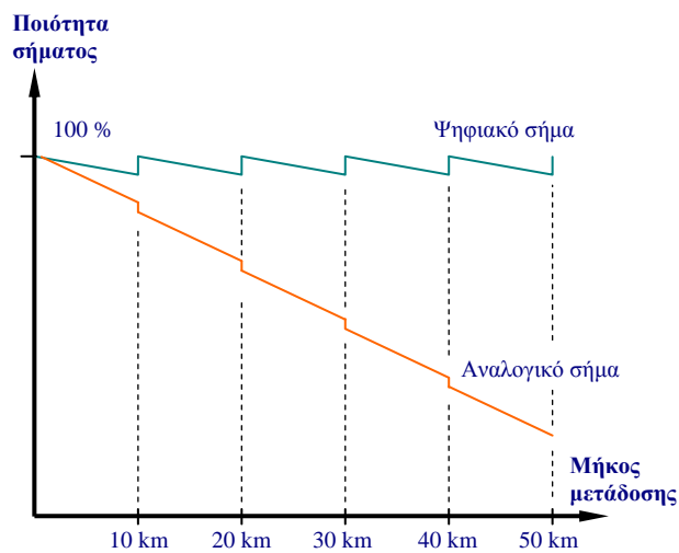
Σχήμα 2.13.1 Η υποβάθμιση της ποιότητας ενός αναλογικού και ενός ψηφιακού σήματος σε σχέση με την απόσταση. Κάθε 10 km υπάρχει αναγεννητής στο ψηφιακό σήμα και ενισχυτής στο αναλογικό. Η ποιότητα στο ψηφιακό στο τέλος παραμένει αμετάβλητη
