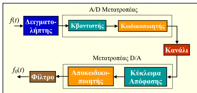
Σχ. 5.8.5. Μπλοκ διάγραμμα ενός πομπού και ενός δέκτη PCM.
