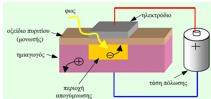
Σχήμα 6.3.2 Ο μικροσκοπικός πυκνωτής που φορτίζεται ανάλογα με το φως που προσπίπτει πάνω του. Ένα CCD μπορεί να έχει στην επιφάνειά του εκατομμύρια τέτοιους πυκνωτές.
