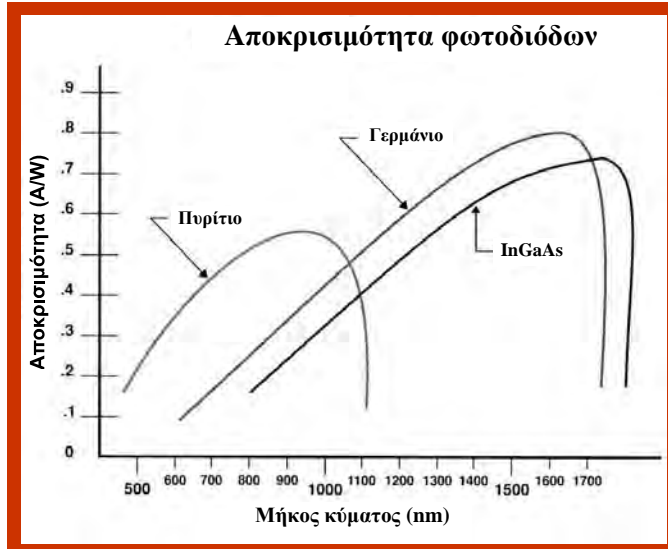
Σχ. 4.5.2. Καμπύλες αποκρισιμότητας φωτοδιόδων συναρτήσει του μήκους κύματος του προσπίπτοντος φωτός για υλικά Si, Ge, InGaAs.
