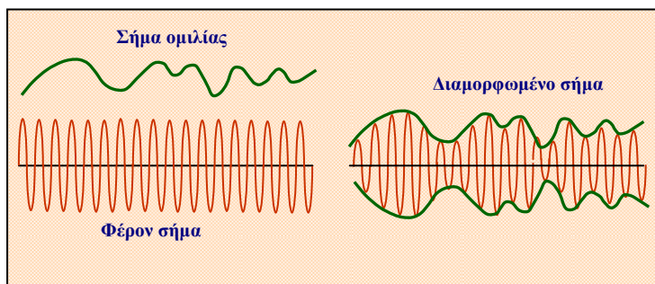
Σχήμα 6.2.1. Διαβίβαση ηλεκτρικού ρεύματος τηλεφωνικής ομιλίας πάνω σε ρεύμα υψηλής συχνότητας (φέρων σήμα).
