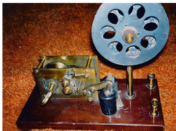
Σχήμα 2.4.7. Καταγραφικό τηλεγράφου του 1860 με χάρτινη ταινία.
