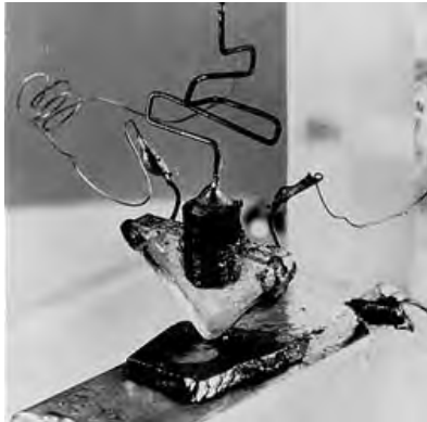
2.12.3. Το πρώτο τρανζίστορ το 1948.
