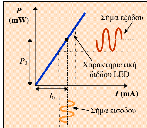
Σχ. 4.4.3. Χαρακτηριστική οπτικής ισχύος εκπομπής - ρεύματος πόλωσης διόδου LED. Η διαμόρφωση του ρεύματος οδήγησης της LED από το σήμα πληροφορίας, μετατρέπονται από το γραμμικό τμήμα της καμπύλης σε αντίστοιχες διακυμάνσεις της οπτικής ισχύος εξόδου.
