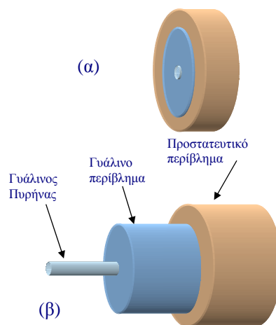
Σχήμα 3.4.2: (α) Τομή οπτικής ίνας, (β) λεπτομέρεια διαστρωμάτωσης οπτικής ίνας.
