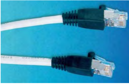
Σχ. 3.1.4. Οι συνδετήρες (RJ45) με τους οποίους τερματίζονται τα καλώδια που περιέχουν χάλκινα ζεύγη.
