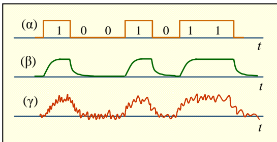
Σχ. 5.4.2. Αλλοιώσεις κυματομορφής σε ψηφιακά συστήματα: (α) Τυπική μορφή ψηφιακών παλμών, (β) Παραμόρφωση κυματομορφής λόγω περιορισμένης χωρητικότητας καναλιού, (γ) Επίδραση προσθετικού θορύβου.
