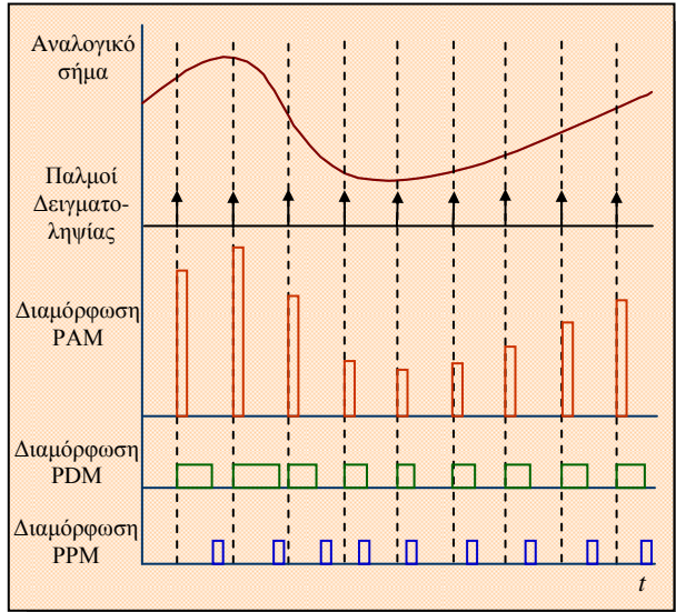
Σχ. 5.7.1. Παλμικές διαμορφώσεις.
