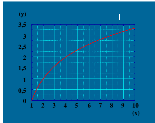
Σχ. 5.3.1. Λογαριθμική συνάρτηση y=\log_2(x) .
