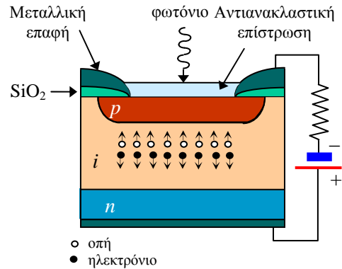
Σχ. 4.5.1. Δομή και συνδεσμολογία μια διόδου PIN.
