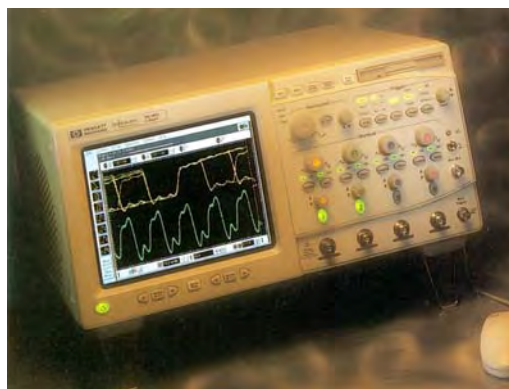
Σχήμα 1.3.2 Ο παλμογράφος απεικονίζει στην οθόνη του μεταβαλλόμενες τάσεις.
