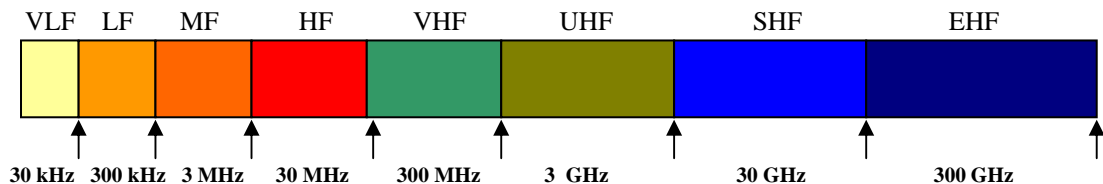
Σχήμα 3.3.2 Οι ζώνες συχνοτήτων και οι ονομασίες τους.
