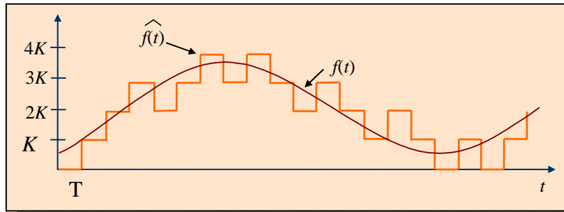
Σχ. 5.8.6. Σήμα πληροφορίας f(t) και η προσέγγισή αυτού \hat{f}(t) .
