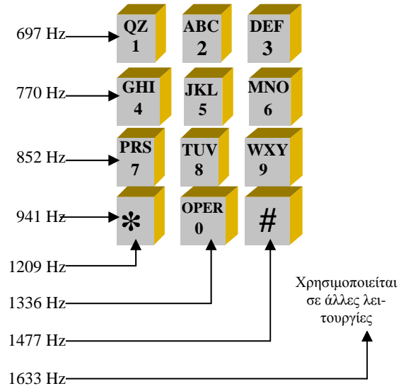
Σχ. 6.1.5 Οι συνδυασμοί συχνοτήτων για την μετάδοση των ψηφίων σε συσκευές με πληκτρολόγιο. Το πλήκτρο «6» π.χ. αντιστοιχεί στις συχνότητες 770 Hz και 1477 Hz.
