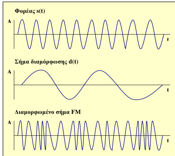
Σχήμα 5.10.5: Διαμόρφωση σημάτων κατά συχνότητα (FM)
