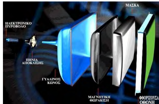
Σχήμα 6.3.5 Τα μέρη του σύγχρονου καθοδικού σωλήνα. Η εκτροπή της ηλεκτρονικής δέσμης γίνεται με μαγνητικό πεδίο από τα πηνία απόκλισης που βρίσκονται εξωτερικά αμέσως μετά το ηλεκτρονικό πυροβόλο.
