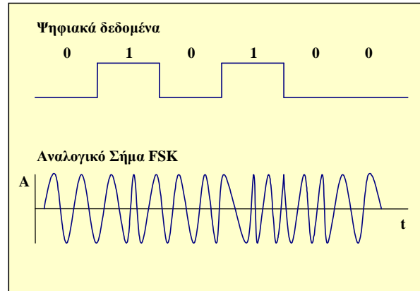
Σχήμα 5.10.8: Διαμόρφωση ψηφιακών σημάτων κατά συχνότητα (FSK)
