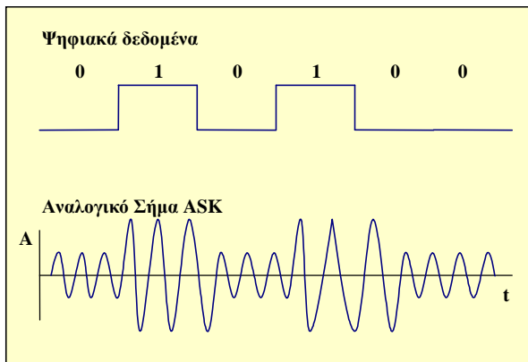
Σχήμα 5.10.7: Διαμόρφωση ψηφιακών σημάτων κατά πλάτος (ASK)
