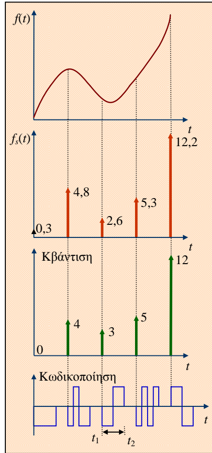
Σχ. 5.8.3. Διαδικασία κβάντισης και κωδικοποίησης. Οι αρνητικοί παλμοί παριστάνουν "0" και οι θετικοί "1".
