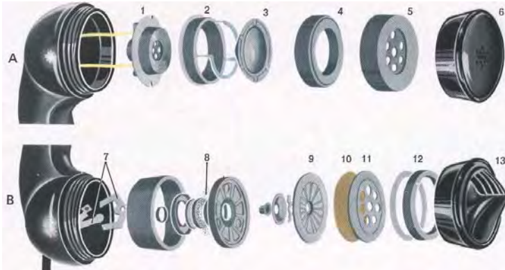
Σχήμα. 6.1.3 Τα εξαρτήματα του μικροτηλέφωνα.
