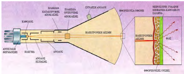
Σχήμα 6.3.4 Ο μονόχρωμος καθοδικός σωλήνας. Στα δεξιά λεπτομέρεια της φθορίζουσας επιφάνειας.
