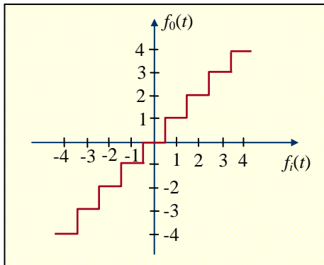
Σχ. 5.8.2. Χαρακτηριστική εισόδου f_i(t) - εξόδου f_o(t) του κβαντιστή του παραδείγματος.
