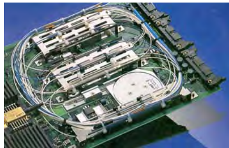
Σχ. 4.6.4. Οπτικός ενισχυτής ίνας. Στο κάτω αριστερό άκρο διακρίνεται το laser άντλησης.
