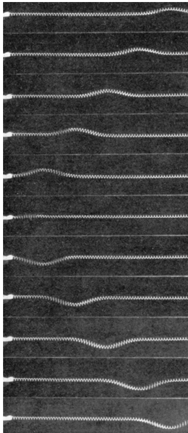
Σχήμα 1.4.1 Κίνηση ενός παλμού σε ελατήριο. Το αριστερό άκρο είναι σταθερό. Οι εικόνες αυτές πάρθηκαν με κινηματογραφική μηχανή σε διαδοχικές χρονικές στιγμές που απέχουν χρονικά 1/24 δευτερόλεπτα. Από αυτές τις εικόνες προκύπτουν μερικά συμπεράσματα σχετικά με την διάδοση:
