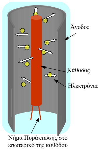
Σχήμα 2.9.3. Η δίοδος λυχνίας στην οποία φαίνεται με βέλη η κίνηση των ηλεκτρονίων από την πυρακτωμένη κάθοδο προς την άνοδο.
