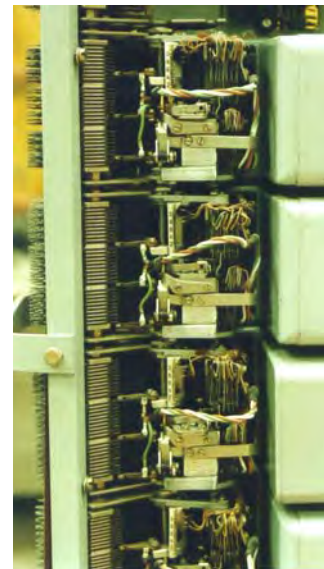
Σχήμα 7.1.5 Οι μηχανισμοί ενός ηλεκτρομηχανικού κέντρου
