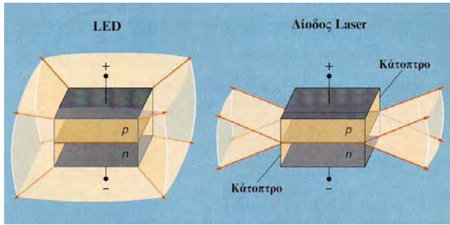
Σχ. 4.4.1. Εκπομπή φωτός από LED και Laser.
