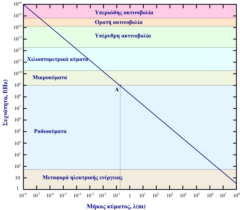
Σχ. 3.3.4. Οι συχνότητες και τα αντίστοιχα μήκη κύματος για τις κυριότερες περιοχές του φάσματος όπως προκύπτουν από τη σχέση c=f \cdot \lambda .
