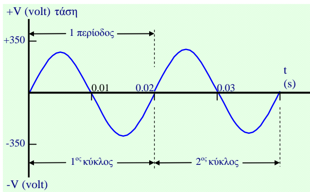
Σχήμα 1.3.1 Γραφική παράσταση της εναλλασσόμενης τάσεως μιας παροχής ηλεκτρικού ρεύματος, όπως απεικονίζεται στον παλμογράφο. Στον οριζόντιο άξονα ο χρόνος μετράται σε δευτερόλεπτα. Η τάση αυτή περιγράφεται και από τη σχέση V=310 \cdot \eta\mu(100 \cdot \pi \cdot t)
