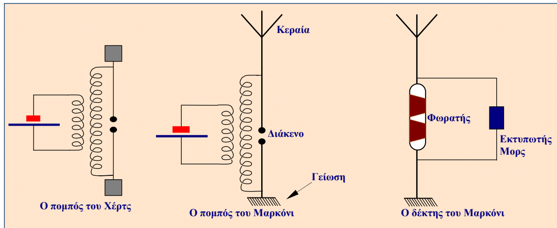
Σχήμα 2.8.4. Ο πομπός και ο δέκτης του Μαρκόνι
