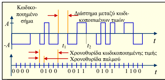
Σχ. 5.8.4. Δυαδική αναπαράσταση των κωδικοποιημένων τιμών με παλμούς και τα τμήματα του χρόνου που αντιστοιχούν στους παλμούς και τις κωδικοποιημένες τιμές.
