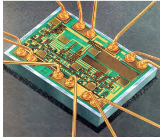
Σχ. 4.2.9. Φωτογραφία ολοκληρωμένου κυκλώματος.
