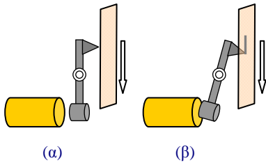
Σχήμα 2.4.4. Όταν ο ηλεκτρομαγνήτης του δέκτη δεν διαρρέετε από ρεύμα(α), η γραφίδα δεν σημειώνει τίποτε. Όταν πιέζεται το πλήκτρο στον πομπό και ο ηλεκτρομαγνήτης διαρρέετε από ρεύμα (β), έλκει την γραφίδα η οποία σημειώνει γραμμή.
