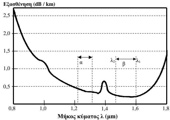
Σχήμα 3.4.6. Παράθυρα χαμηλής εξασθένησης στις μονότροπες οπτικές ίνες.
