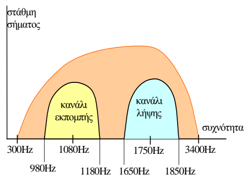
Σχήμα 6.4.3. Ο διαχωρισμός του καναλιού ομιλίας σε δύο τμήματα (κανάλια). Το αριστερό χρησιμοποιείται από το μόντεμ που κάλεσε.
