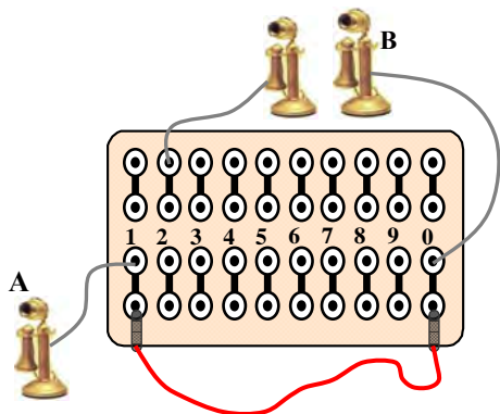
Σχήμα 7.1.3 Η σύνδεση δύο συνδρομητών στο μεταλλάκτη του χειροκίνητου κέντρου. Η σύνδεση του Α και του Β γίνεται με το κόκκινο συνδετικό καλώδιο.
