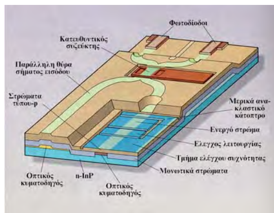
Σχ. 4.7.3. Σχηματικό διάγραμμα ολοκληρωμένου οπτικοηλεκτρονικού φωτοδέκτη.
