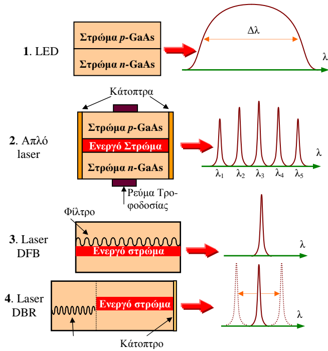
Σχ. 4.4.10. Μήκη κύματος εκπομπής διόδων laser και LED.
