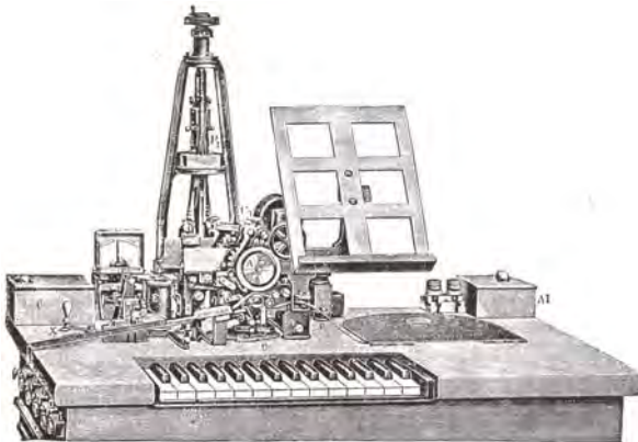
Σχ. 2.4.8. Εκτυπωτικός τηλεγράφος του Χιουζ. Στον τηλεγράφο αυτό, δύο τροχοί ένας σε κάθε σταθμό εκπομπής και λήψης, έφεραν στην περιφέρειά τους ανάγλυφα τα ψηφία του αλφαβήτου και περιστρέφονταν σύγχρονα. Έτσι, όταν ο τροχός του ενός μηχανήματος παρουσίαζε στο κάτω του μέρος λ.χ. το Α, το ίδιο συνέβαινε και στη λήψη. Αν πιεζόταν πάνω στον τροχό εκείνη τη στιγμή, μια χάρτινη ταινία θα τυπωνόταν επάνω της το σύμβολο Α.
