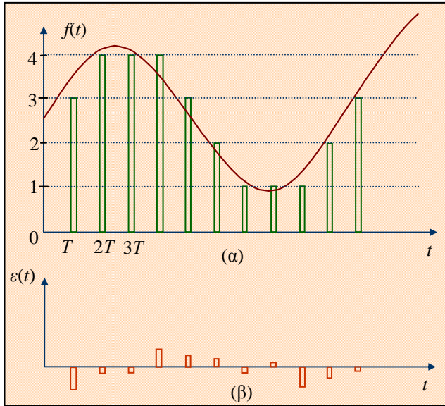
Σχ. 5.8.1. (α) Διαδικασία της κβάντισης, (β) το σφάλμα της κβάντισης.
