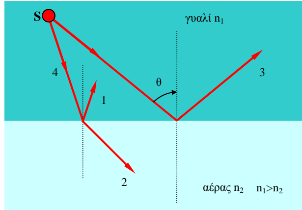
Σχήμα 3.4.1. Οι ακτίνες της πηγής S κατευθύνονται από μέσο με μεγάλο δείκτη διάθλασης (δ.δ.), σε μέσο με μικρό δ. δ.
