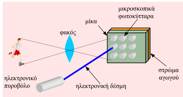
Σχήμα 6.3.1 Αρχή λειτουργίας της εικονοληπτικής λυχνίας.
