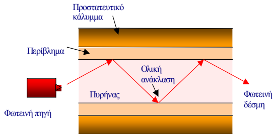
Σχήμα 3.4.3. Ο μηχανισμός διάδοσης στην οπτική ίνα
