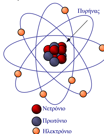
Σχήμα. 1.1.1 Σύμφωνα με το μοντέλο του Μπορ τα αρνητικά ηλεκτρόνια περιστρέφονται γύρω από τον θετικό πυρήνα. Το ηλεκτρόνιο έχει φορτίο -1,6 \cdot 10^{-19} C. Το νετρόνιο είναι ουδέτερο ενώ το πρωτόνιο έχει φορτίο +1,6 \cdot 10^{-19} C.
