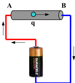
Σχήμα. 1.1.3 Ένα φορτίο q μετακινείται μέσα από τον αγωγό AB παράγοντας έργο W . Η ηλεκτρική πηγή (μπαταρία) παρέχει αυτήν την ενέργεια
