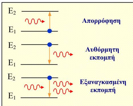
Σχ. 4.4.2. Βασικές αλληλεπιδράσεις ύλης – ενέργειας.
