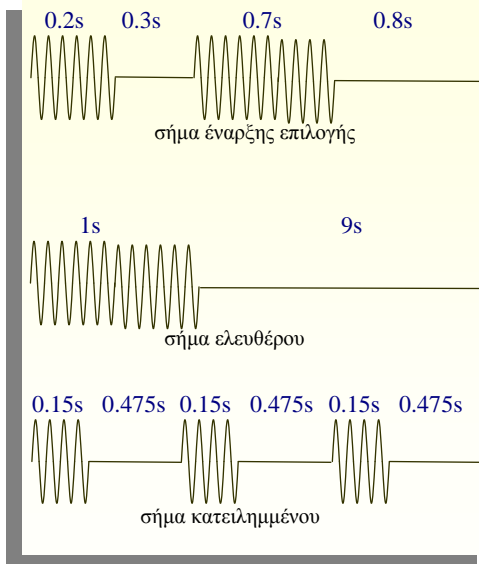
Σχήμα 7.3. Οι διάρκειες των (ηχο)σημάτων
