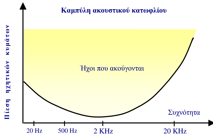
Σχήμα 6.1.2 Στο διάγραμμα κατωφλίου ακουστότητας η γραμμοσκιασμένη περιοχή δείχνει τους ήχους που αντιλαμβάνεται το ανθρώπινο αυτί. Η κλίμακα στις συχνότητες δεν είναι γραμμική. Το ανθρώπινο αυτί μπορεί να ακούσει ήχους με συχνότητες από 20 Hz μέχρι 20.000 Hz (ή 20KHz). Η παραπάνω περιοχή συχνοτήτων (ή φάσμα) ονομάζεται ακουστικό φάσμα.
