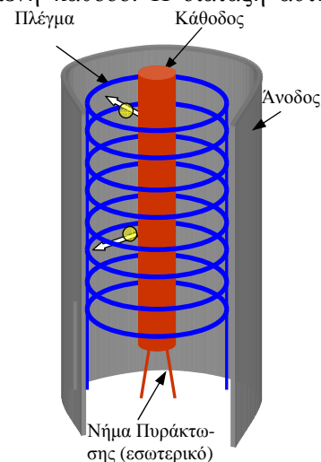
Σχήμα 2.9.4. Η τριόδος λυχνία περιλαμβάνει το πλέγμα. Τα ηλεκτρόνια για να φτάσουν στην άνοδο είναι υποχρεωμένα να περάσουν μέσα από το πλέγμα. Έτσι ελέγχεται το ρεύμα ανόδου - καθόδου.
