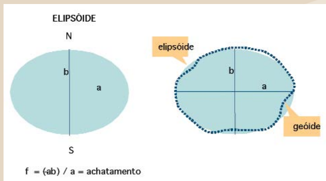
Figura 4. Representação do elipsóide e do geóide.
