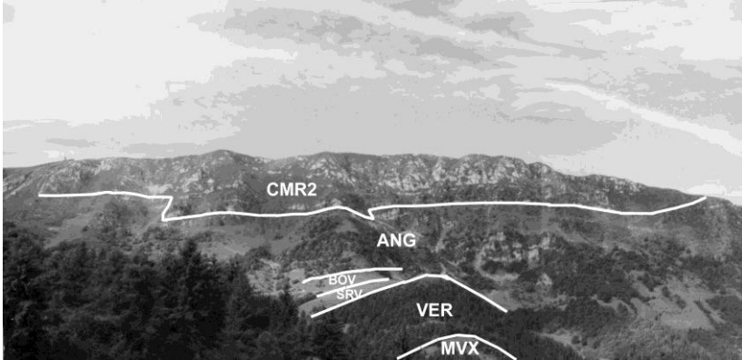
Fig. 5 – Panoramica della dorsale del Monte Guglielmo vista da N (MVX= Micascisti a clorite e mica chiara; VER= Verrucano Lombardo; SRV= Servino; BOV= carniola di Bovegno; ANG= Calcarea di Angolo; CMR 2 = membro del Calcarea di Monte Guglielmo).
