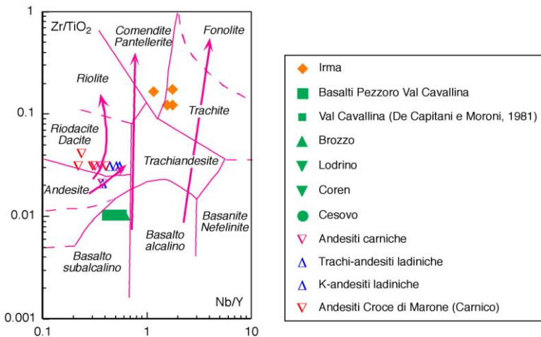
Fig. 7 - Diagramma Zr/TiO_2-Nb/Y (WINCHESTER & FLOYD, 1977) per le vulcaniti ladinicke e carniche della regione Bresciana del F. Iseo.
