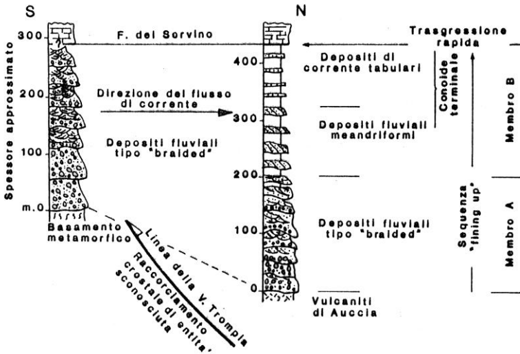
Fig. 3 – Caratteristiche dei depositi del Verrucano Lombardo affioranti tra la dorsale tromplina (a sinistra) ed il bacino di Collio (a destra).
