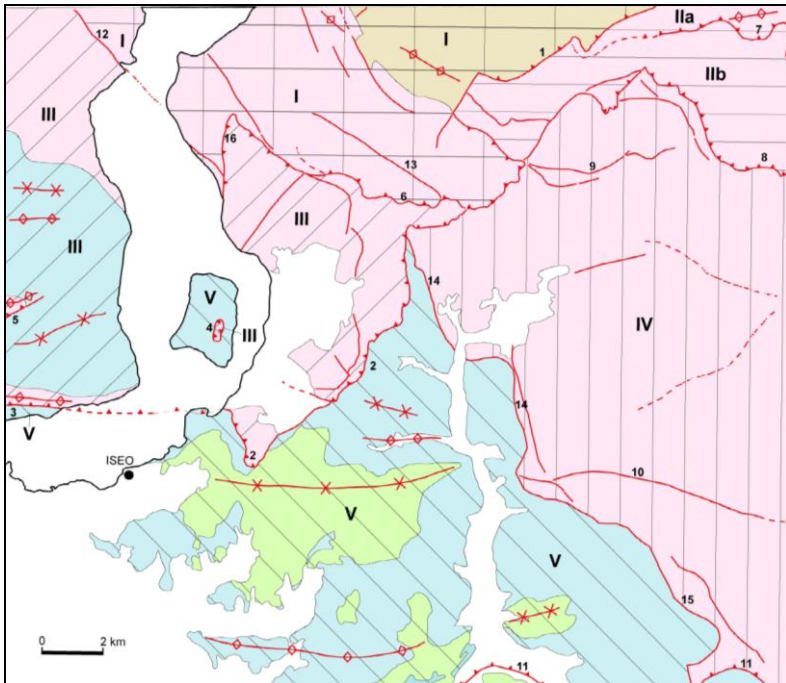
Fig. 20 – Schema strutturale del Foglio Iseo
