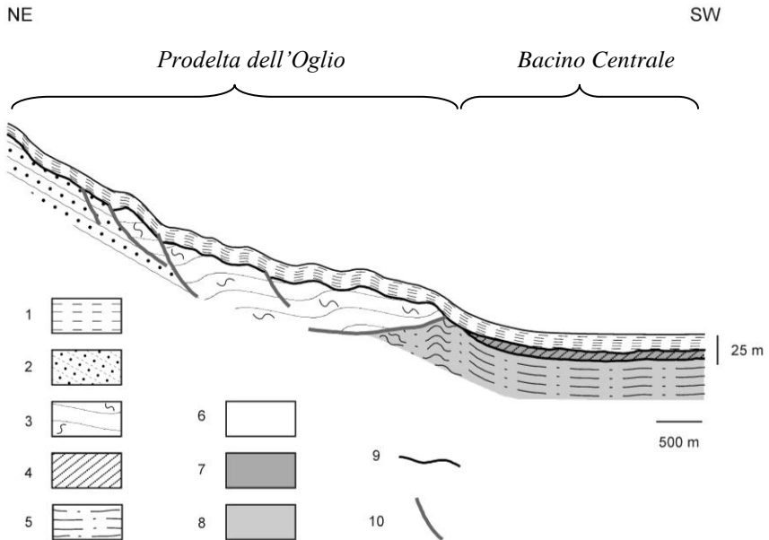
Fig. 19 - Relazioni stratigrafiche tra le unità riconosciute nella parte N del Lago d'Iseo. 1 = sedimenti lacustri (SEQUENZA A), 2 = depositi alluvionali, 3 = accumuli gravitativi, 4 = depositi glaciali (SEQUENZA B), 5 = depositi lacustri (SEQUENZA C); età relative dei depositi: 6 = post-LGM, 7 = LGM, 8 = pre-LGM; 9 = unconformities, 10 = superfici di scivolamento.
