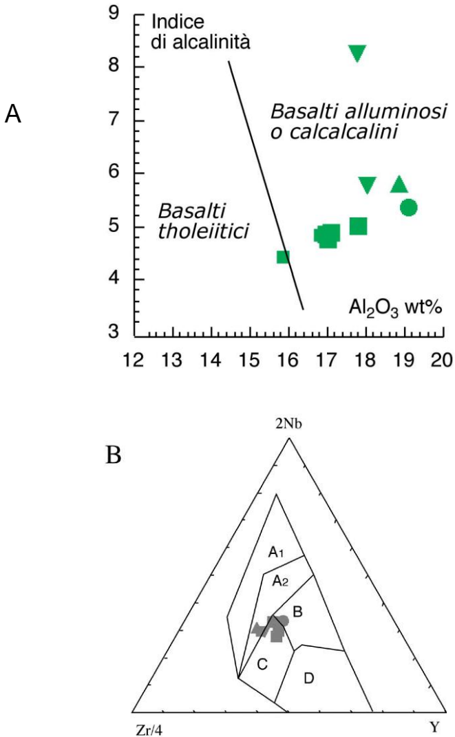
Fig. 9 - (A) Indice di alcalinità (MIDDLEMOST, 1975) vs. \text{Al}_2\text{O}_3 e (B) diagramma 2Nb-Zr/4-Y (MESCHÉDE, 1986) per i basalti triassici del F. Iseo. A 1 : basalti alcalini intraplacca, A 2 : basalti alcalini e tholeiitici intraplacca; (B): E(nriched)-type MORB (basalti di dorsale oceanica arricchiti), C: tholeiitici intraplacca e basalti di arco vulcanico, D: N(ormal)-type MORB (basalti di dorsale oceanica normali) e basalti di arco vulcanico.
