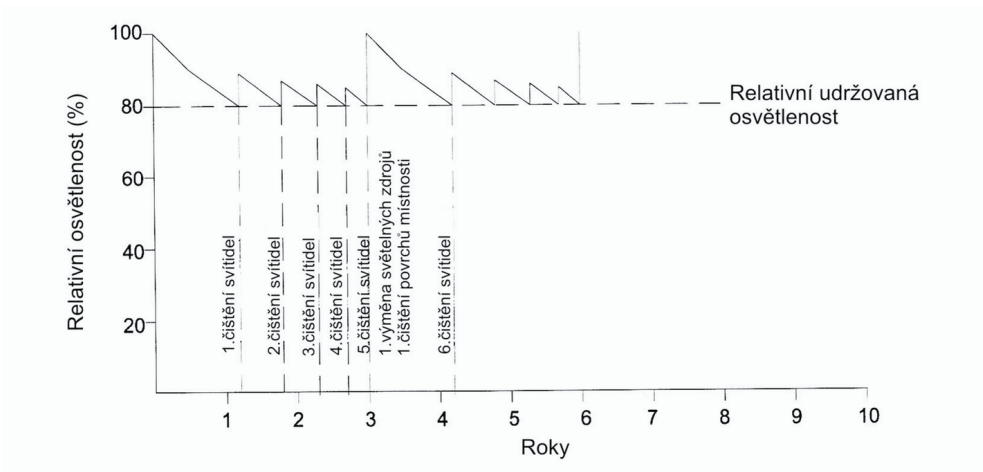
Obr. 12.4: Plán údržby s proměnným intervalem čištění [11]
