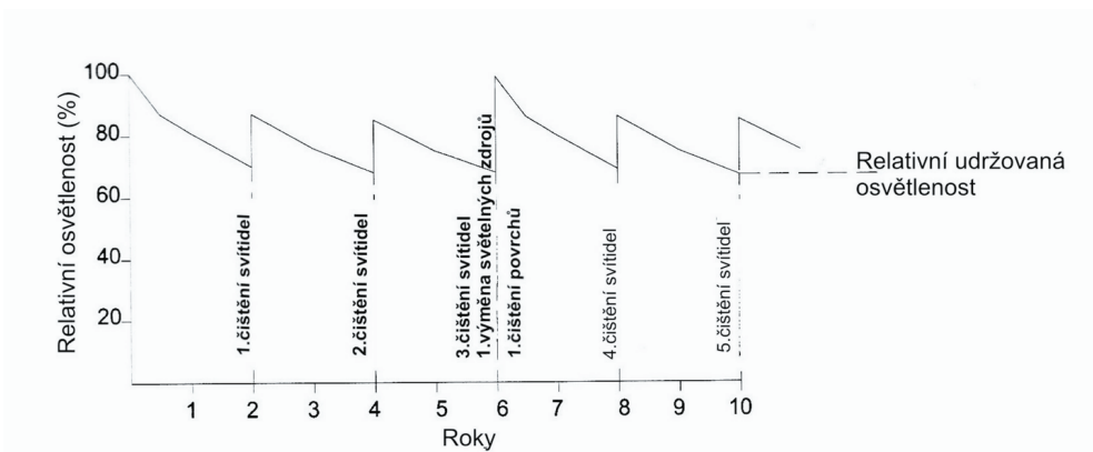
Obr. 12.3: Plán údržby se stálým intervalem čištění [11]
