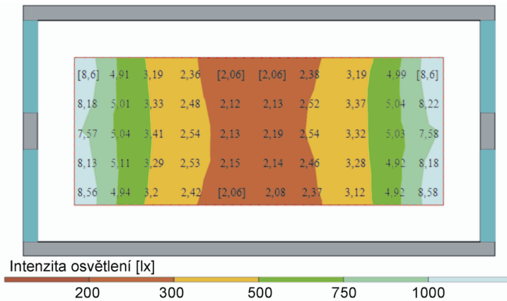
Obr. 5.8: Rozložení osvětlenosti v místnosti a D u dvoustranné boční osvětlovací soustavy
