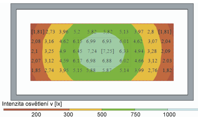
Obr. 5.9: Rozložení osvětlenosti v místnosti u horní osvětlovací soustavy
