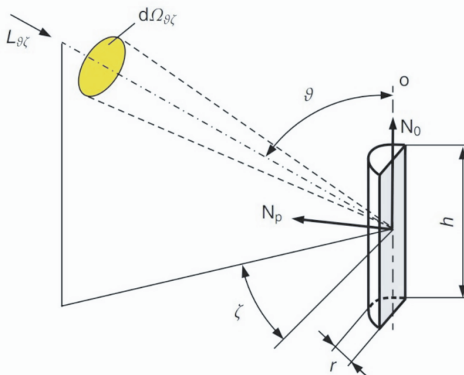
Obr. 2.23: Poloválcová osvětlenost [3]
