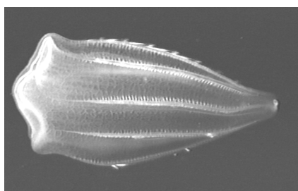
Fig. 30. Beroë ovata
