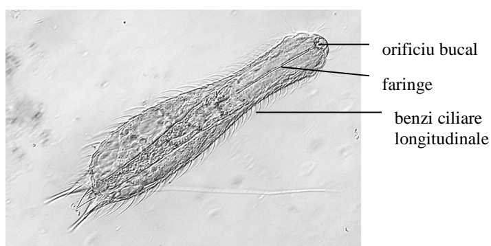
Fig. 41. Chaetonotus maximus
