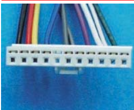
PC3-453- Anschlußkabel f. Orig. KENWOOD 11pol/ISO
