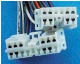
PC3-213- Anschlußkabel für Original VOLVO OEM ab 9/94 auf lose Enden.
