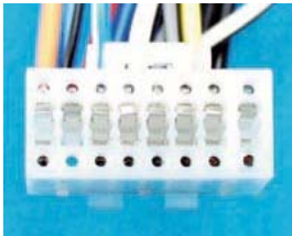
PC3-485- Anschlußkabel f. Orig. DENON 16pol/ISO
