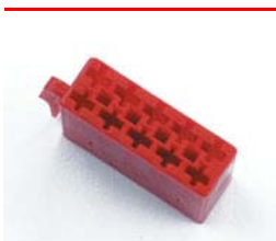
18069 10 pol. ISO Buchse 10 Stk. lose Erklärungen: Die Bezeichnung Buchse und Stecker wird bei ISO vom Kontaktmaterial abgeleitet. Bestückung mit weibl. Doppelfederkontakt 18068.
