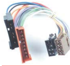
19634 ISO -> FORD, JAGUAR S-Type ab 99 24 Stk. Inhalt 24 Stück von 19434.
