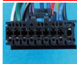
PC3-432- Anschlußkabel f. Original SONY 18pol/ISO
