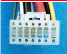
PC3-454- Anschlußkabel f. Orig. KENWOOD 14pol/ISO kleiner Stecker
