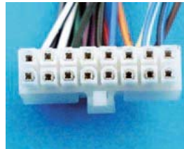
PC3-471- Anschlußkabel f. Orig. CLARION 16pol/ISO
