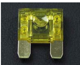
23051 Maxi Sicherung 20 A Vergoldete MAXI Sicherung für alle MAXI Sicherungshalter der GOLD LINE Serie und PROFESSIONAL LINE Serie.
