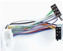
19437 ISO -> HONDA ab 1/99
