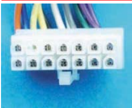
PC3-452- Anschlußkabel f. Orig. KENWOOD 14pol/ISO großer Stecker
