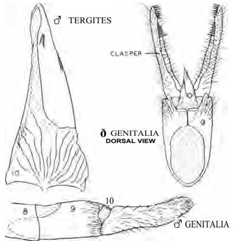
Fig. 34.— Polytrichia xena
