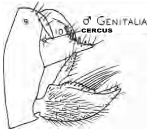
Fig. 118.-- Lepidostoma pleca
