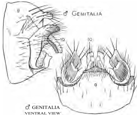
Fig. 110. Neophylax stollus
