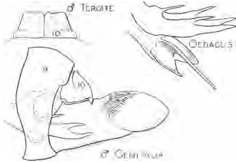
Fig. 6. Rhyacophila mullis
