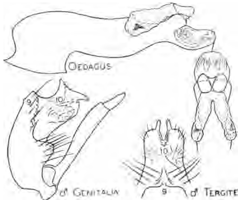
Fig. 83.-- Hydropsyche tana
