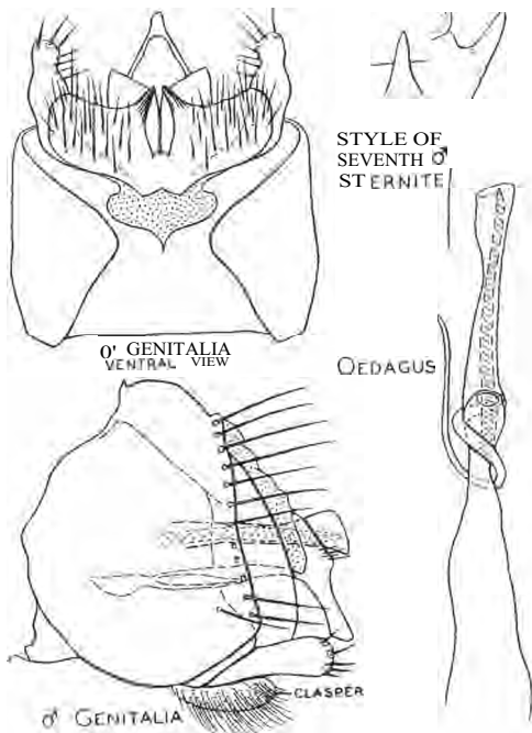
Fig. 21.— Agraylea saltseae
