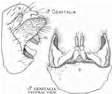
Fig. 109.— Neophylax ayanus
