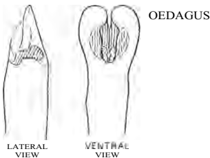
Fig. 67.— Hydropsyche bidens
