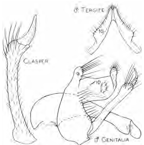
Fig. 85. Cheumatopsyche campyla
