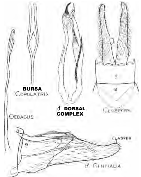
Fig. 30.— Polytrichia shawnee
