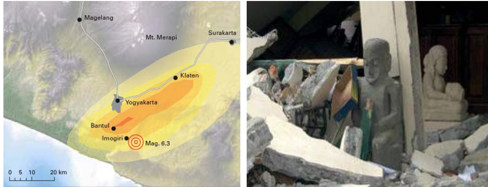
Figura 7.4 Localización del epicentro del sismo del 27 de mayo de 2006 en Indonesia
