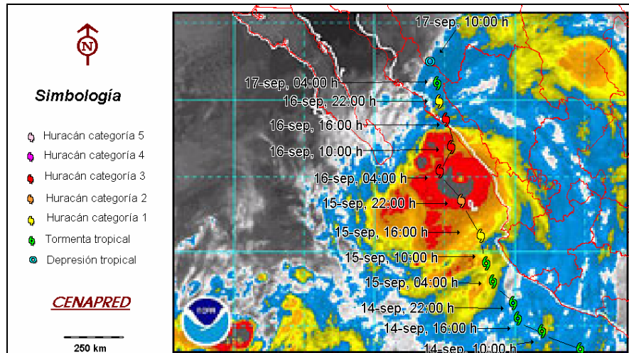
Figura 2.91 Imagen de satélite del huracán Lane aproximándose a la costa de Sinaloa
