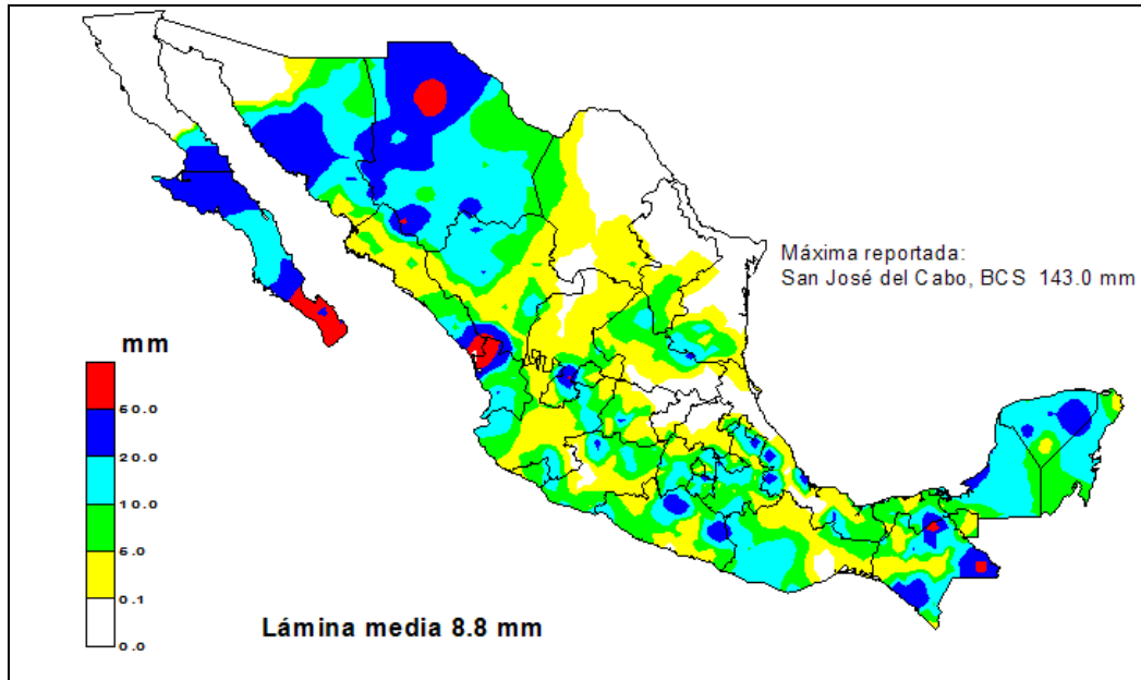
Figura 2.51 Precipitación del 1° de septiembre
