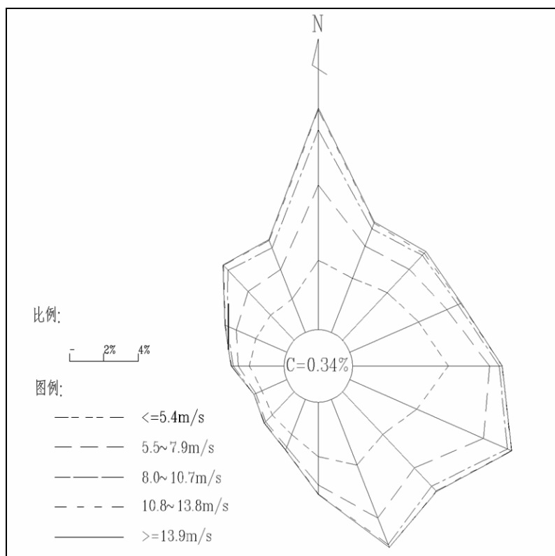
图 4.1-1 风玫瑰图
