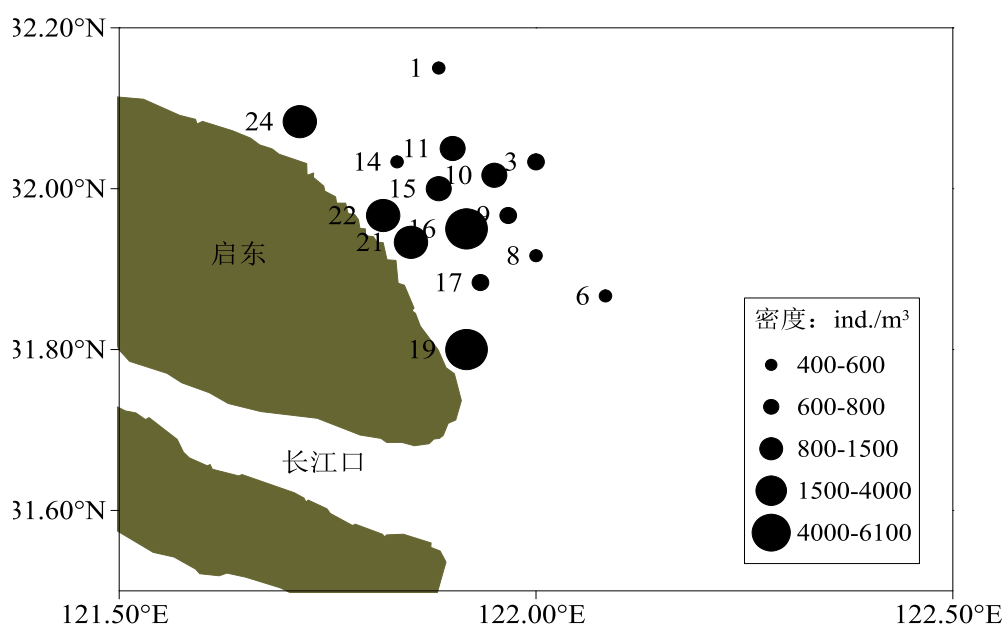
图 5.6-23 2019 年 10 月调查海域各站位 II 型网采浮游动物密度
