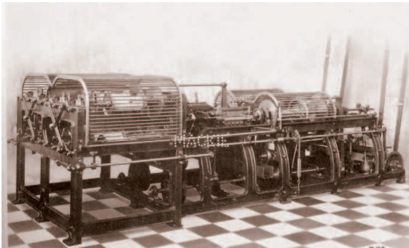
Σχοινοποιητική μηχανή της μεσοπολεμικής περιόδου. Δημοσιεύτηκε από την Ευαγγελία Βαρέλλα
