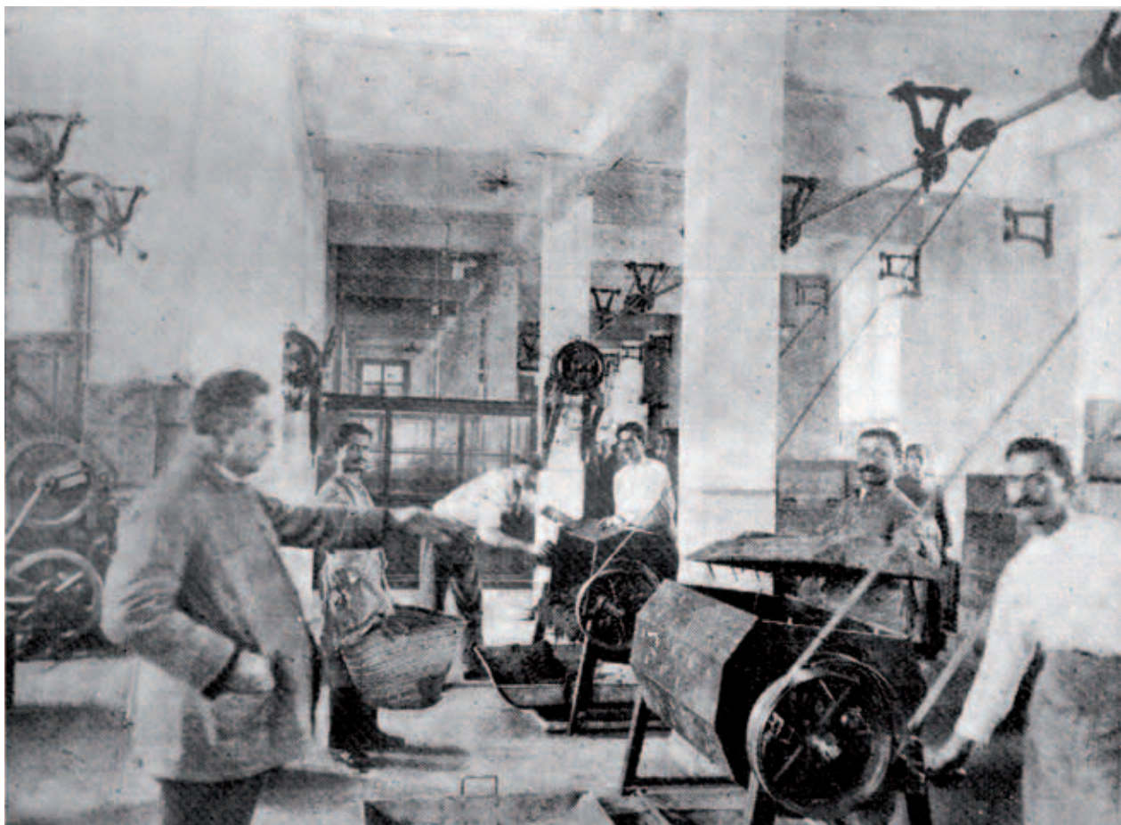
Μηχανήματα τριβής καπνού. Γ. Χατζηϊωάννου. Λεύκωμα Εκατονταετηρίδας
