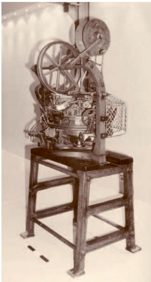
Καλτσομηχανή της μεσοπολεμικής περιόδου. Δημοσιεύτηκε από την Ευαγγελία Βαρέλλα
