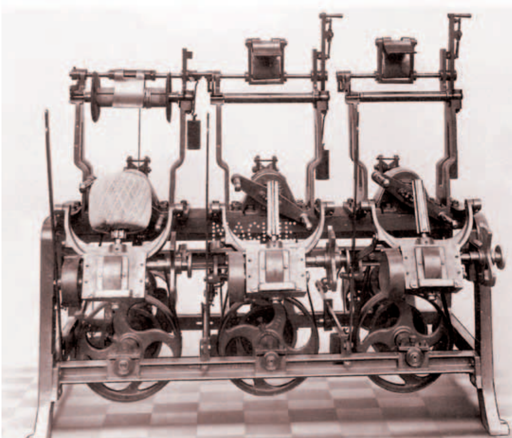
Κουβαρίστρα δεκαετίας 1930. Δημοσιεύτηκε από την Ευαγγελία Βαρέλλα
