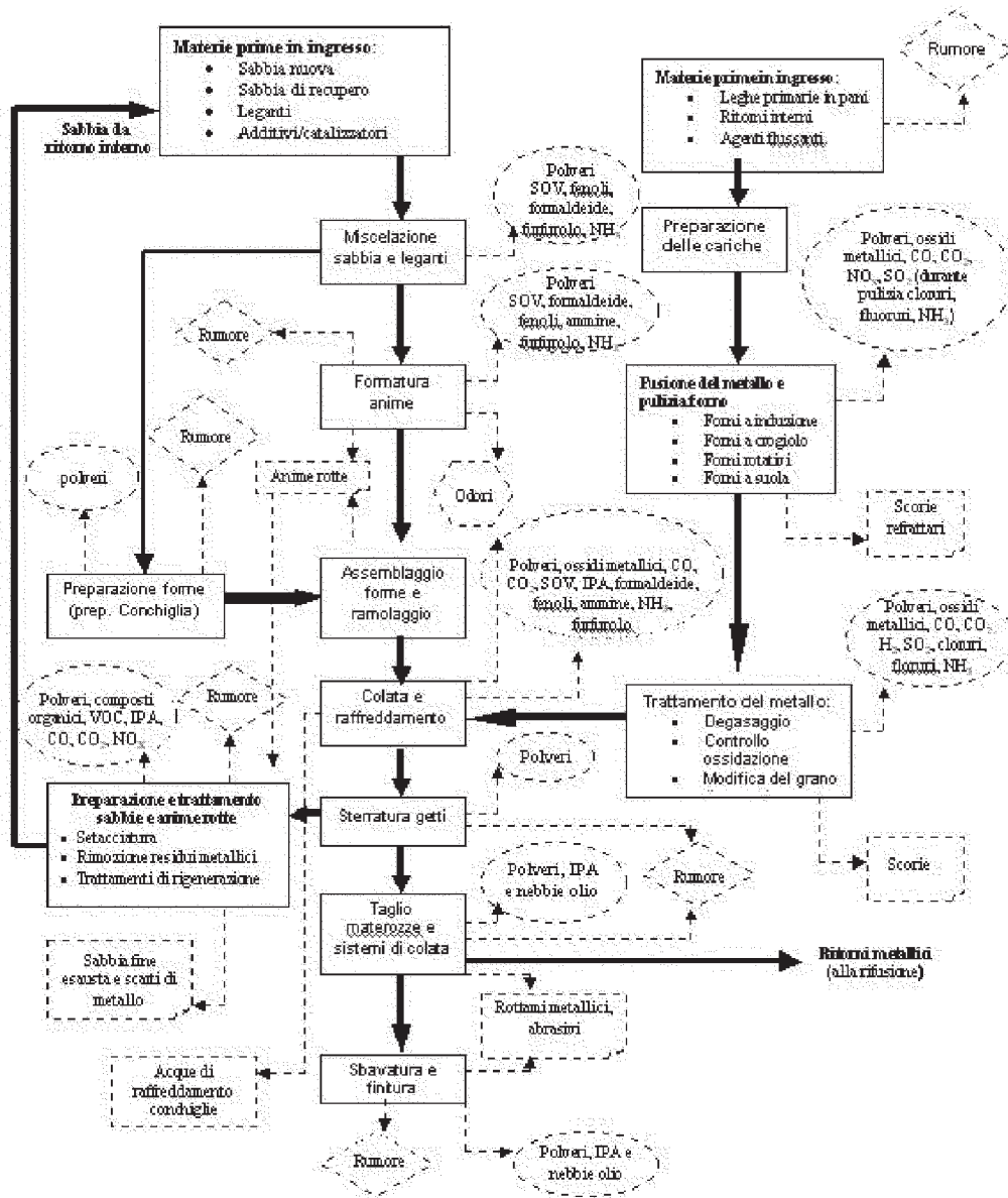
Flusso di processo tipico di una fonderia in sabbia e con colata in forma permanente (metodo di colata a bassa pressione od a gravità)
