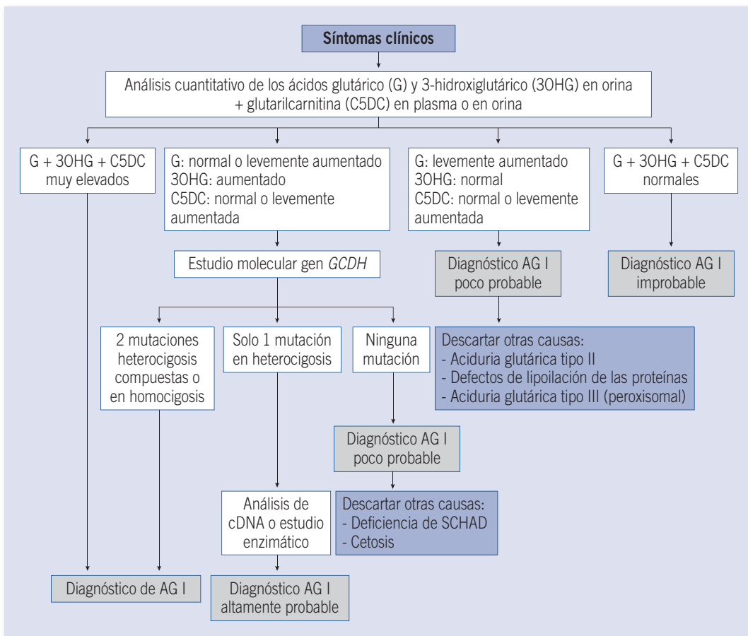
FIGURA 2. Algoritmo diagnóstico.
