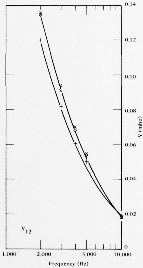
(d) Y_{12} versus frequency.
