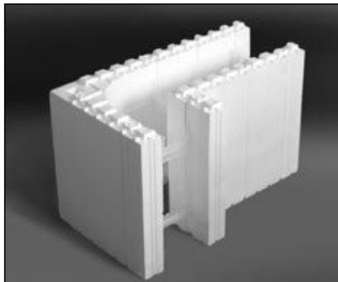
Рис. 7.26. Левый и правый угловые элементы под 90 градусов
