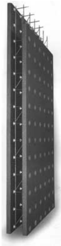
Рис. 7.51. Арматура в несъемной опалубке
