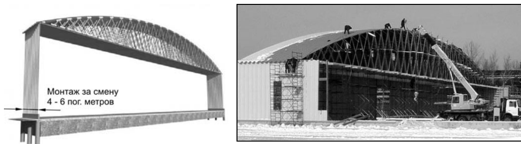
Рис. 5.12. Монтаж несущих конструкций бескаркасного здания
