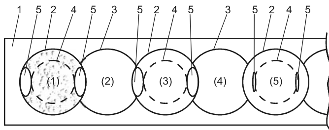
Рис. 3.14. Бурение четных скважин с использованием образованных в нечетных сваях пазов в качестве направляющих, их армирование и бетонирование в них четных свай. Форшахта 1 с направляющими отверстиями для нечетных 2 и четных 3 скважин, каркасы арматуры 4, гибкие армированные рукава 5
