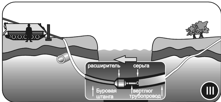
Рис. 2.8. Протягивание трубопровода
