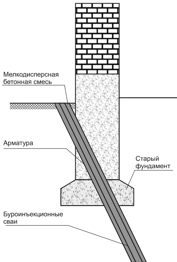
Рис. 3.17. Буроинъекционные сваи
