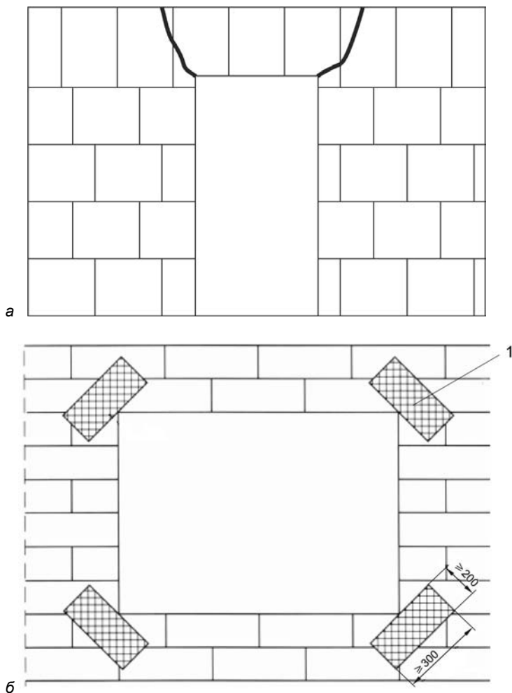
Рис. 7.77. Деформационные трещины в углах дверных и оконных проемов (а) и их предупреждение путем усиления (б) армирующими сетками из стекловолокна; 1 — армирующие сетки
