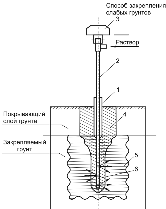
Рис. 4.12. Стадия инъецирования:
