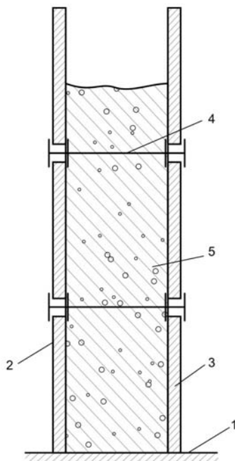
Рис. 7.47. Опалубка из древесно-минеральных материалов: 1 — технологический горизонт; 2 и 3 — внешние и внутренние отдельные щиты опалубки из древесно-минеральных материалов; 4 — гибкие связи; 5 — бетонная смесь
