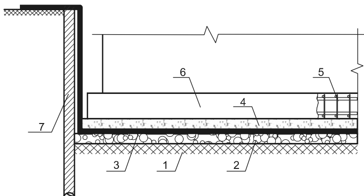
Рис. 4.15. Способ гидроизоляции подземной части здания и сооружения:
