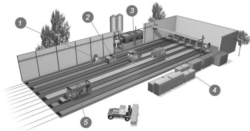
Рис. 7.66. Линия Тенсиланд
