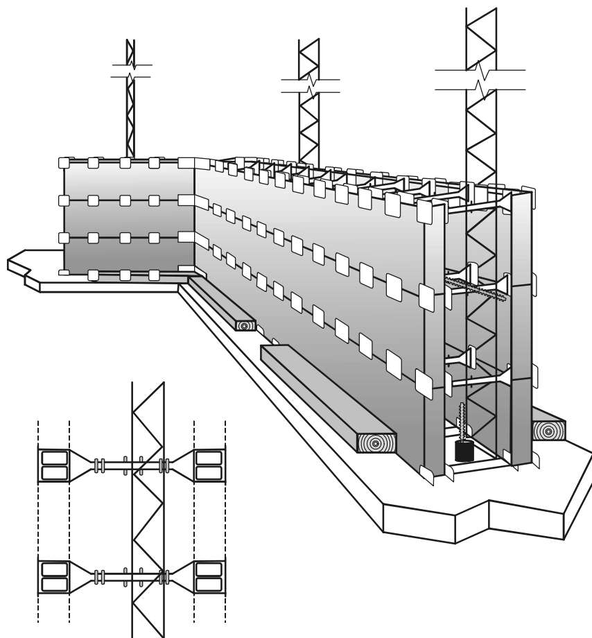
Рис. 7.41. Установка опалубки и арматуры первого яруса бетонирования (стойки и горизонтальные прогоны крепления не показаны)
