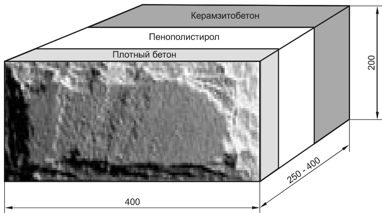
Рис. 7.78. Блок Теплостен
