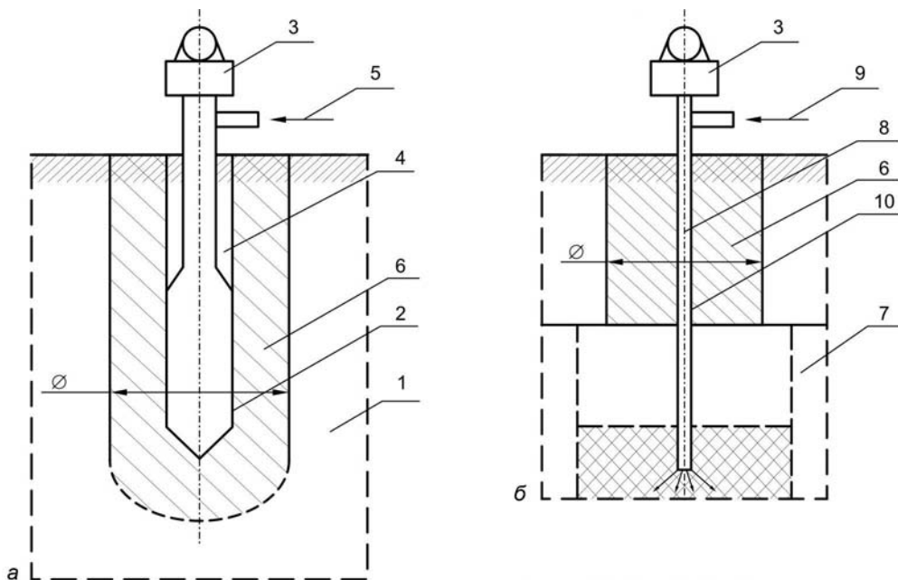
Рис. 4.7. Закрепление водонасыщенных грунтов с одновременной подачей виброшаблона и наполнителя в полость (а), подача иньектора и иньектирование через материал формирующейся цемента-грунтовой сваи (б): 1 — переувлажненный глинистый грунт; 2 — шаблон; 3 — вибратор; 4 — вертикальная или наклонная полость; 5 — песчано-цементная смесь; 6 — формируемая свая; 7 — слабые просадочные грунты; 8 — иньектор; 9 — твердеющий раствор; 10 — контакт
