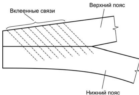
Рис. 4.22. Схема опорного узла линзообразной фермы
