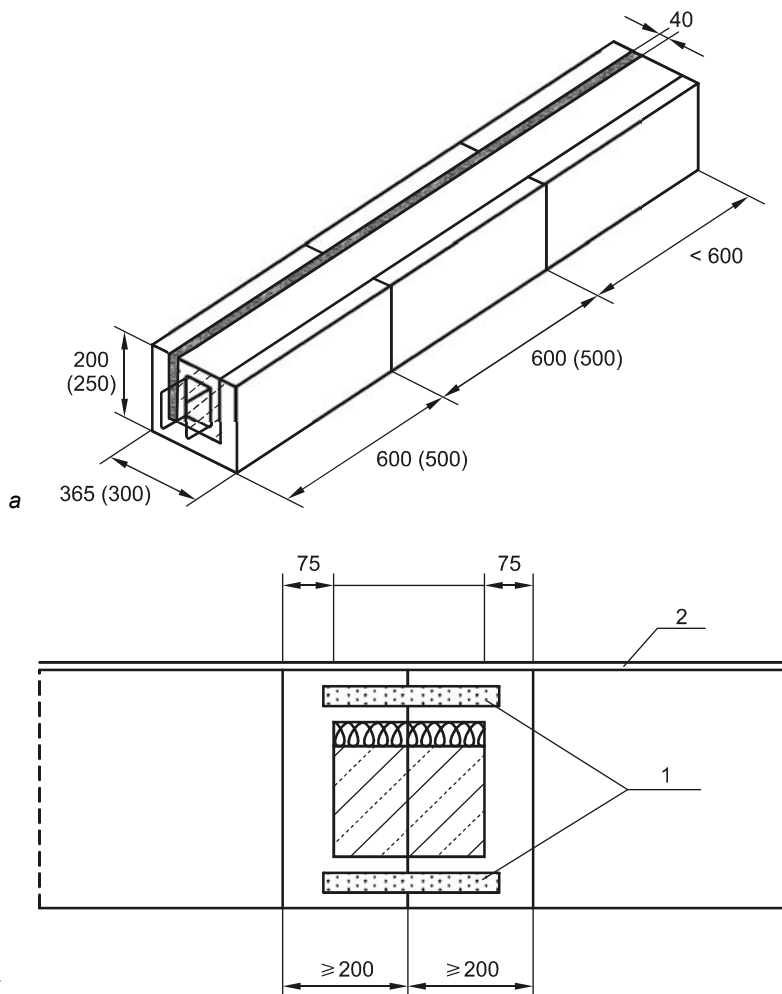
Рис. 7.74. Железобетонные перемычки (а) и простенки (б), изготавливаемые из монолитного железобетона в опалубке из корытообразных пенобетонных элементов: 1 — металлические соединительные пластины; 2 — штукатурный слой
