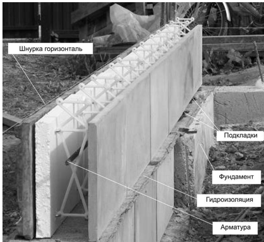
Рис. 7.82. Конструкция техноблока
