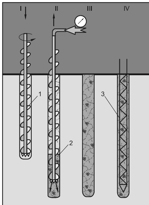
Рис. 3.12. Технологическая схема устройства свай микро CFA:
