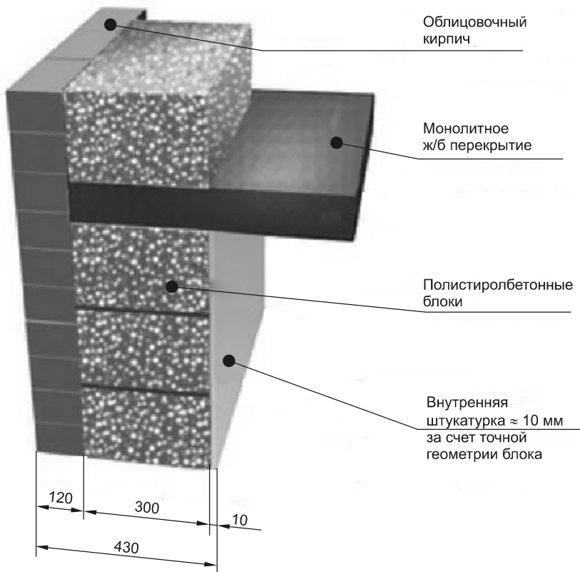
Рис. 7.69. Конструктивная схема
