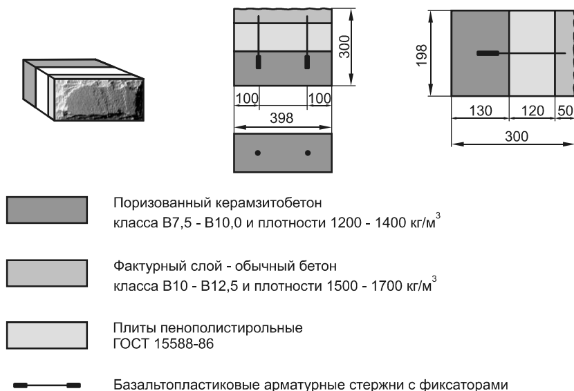
Рис. 7.80. Блок рядовой
