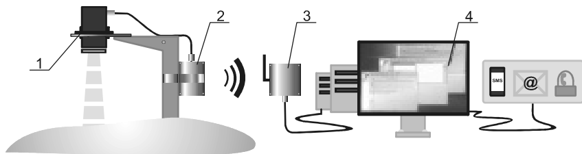
Рис. 6.21. Компоненты системы: 1 — датчик дистанции; 2 — блок управления датчиком дистанции; 3 — блок сбора информации; 4 — промышленный компьютер
