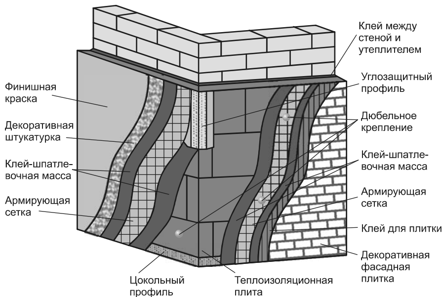
Рис. 7.19. Система утепления фасадов Sarpatect
