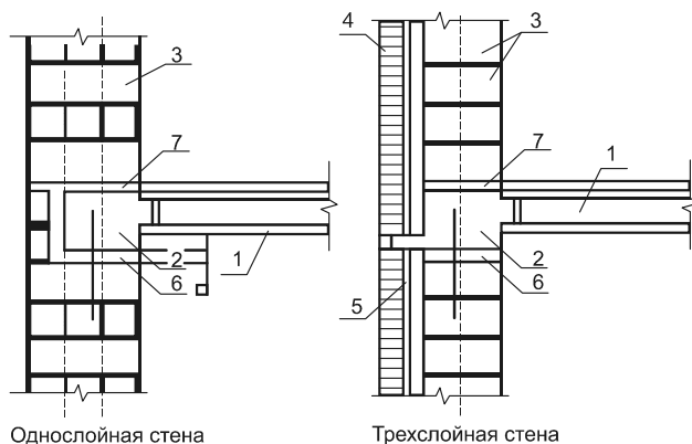
Однослойная стена
