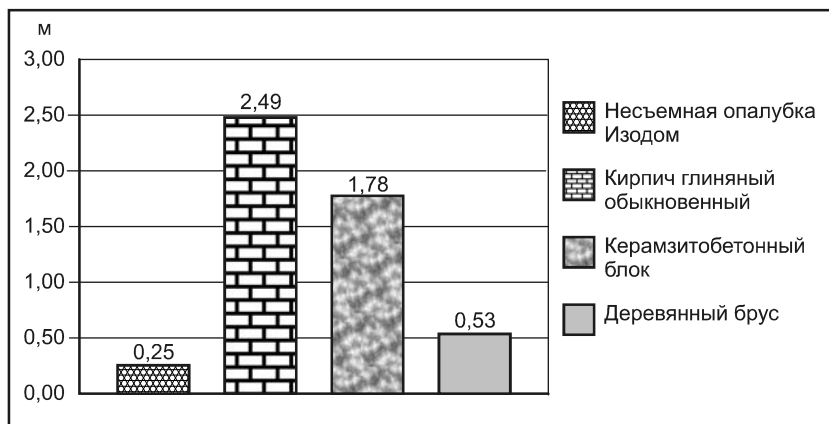
Рис. 7.30. Сравнение по теплосбережению толщины стены из различных материалов
