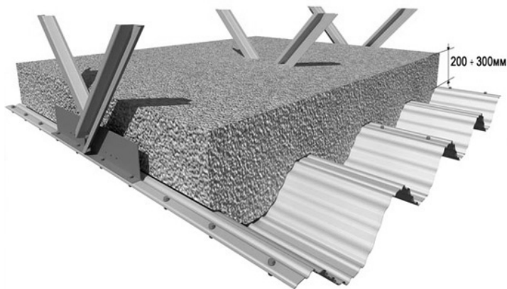
Рис. 5.11. Конструкция покрытия
