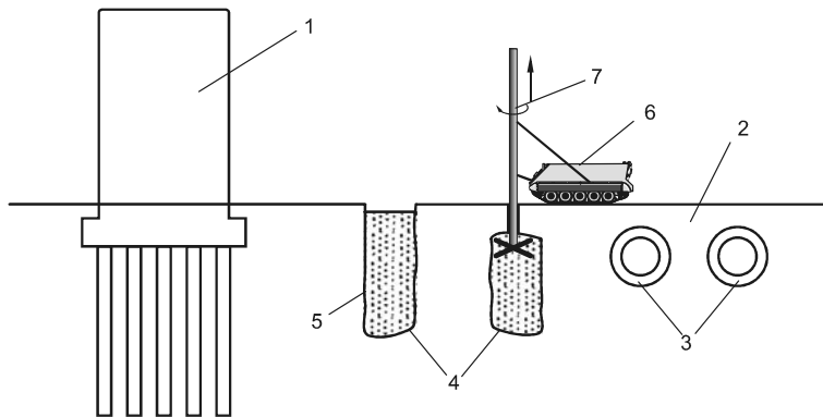
Рис. 8.5. Принципиальная схема: 1 — здание; 2 — грунтовый массив; 3 — источник вибрации; 4 — ряд скважин; 5 — аэрированная водогрунтовая пульпа; 6 — буровая установка; 7 — многотрубная штанга
