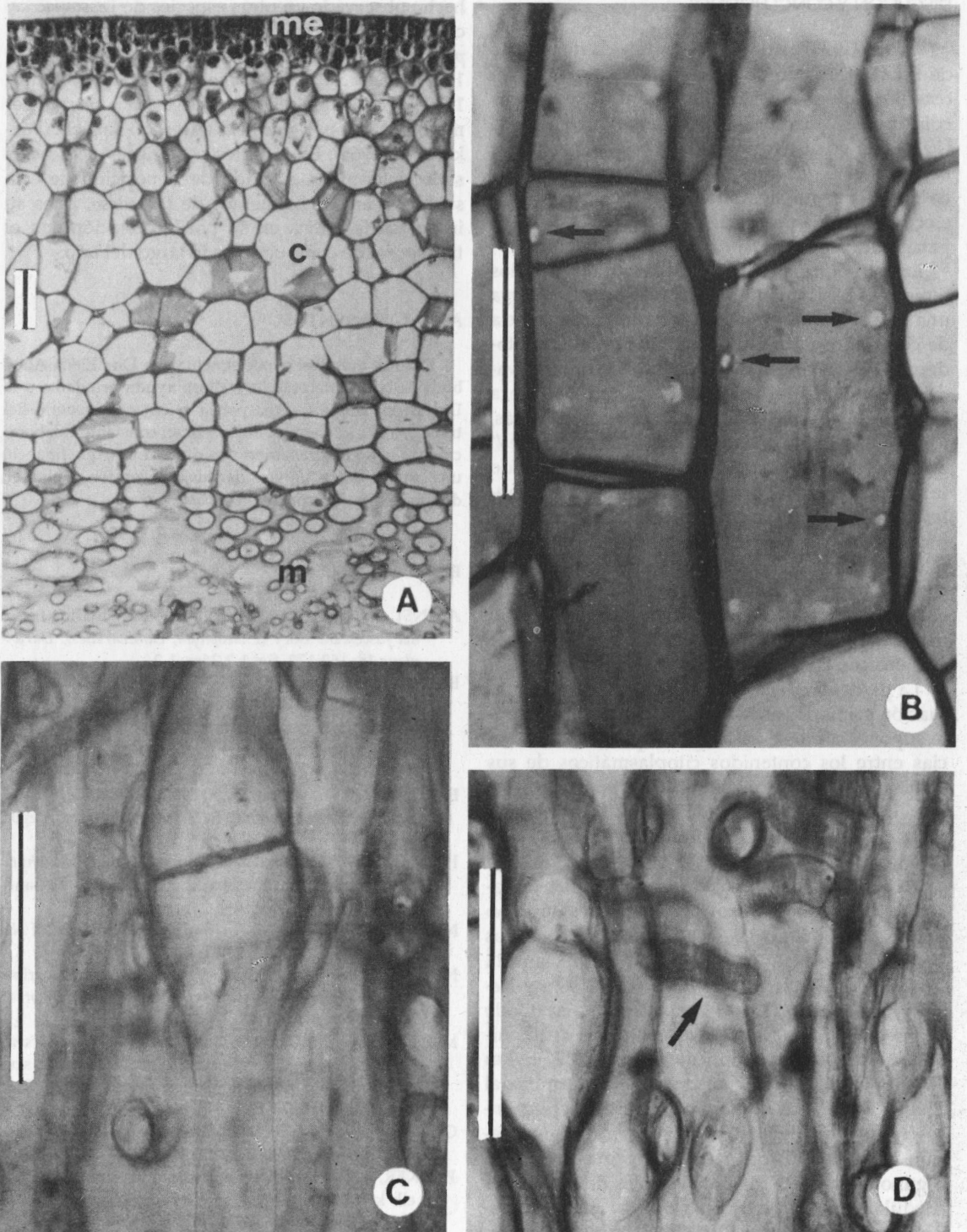
Fig. 3.— A: Corte transversal de filoide, mostrando meristodermo (me), corteza (c) y médula (m). B, C y D: Corte longitudinal de filoide. B: Células corticales, mostrando campos de puntuación primarios (flechas). C: Filamento trompeta de la médula. D: Conexión lateral entre 2 filamentos de la médula (flecha). Escalas: 50 \mu m.
