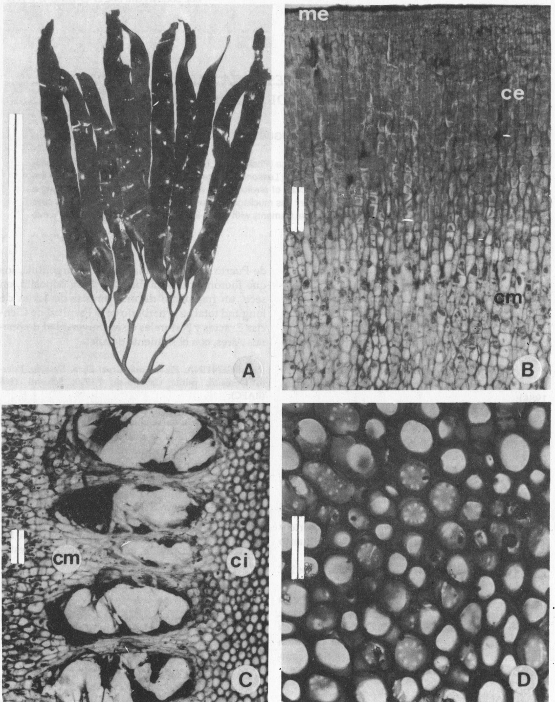
Fig. 1.- A: Vista general de un fragmento de una planta de 1,5 m de largo total. B, C y D: Corte transversal de rama. B: meristodermo (me) con "cutícula", corteza externa (ce) y corteza media (cm). C: Cavidades con mucílago de la corteza media (cm) más corteza interna (ci). D: Corteza interna, mostrando campos de puntuación primarios dispuestos periféricamente en paredes transversales. Escalas: 40 cm (A), 100 µm (B-C) y 50 µm (D).
