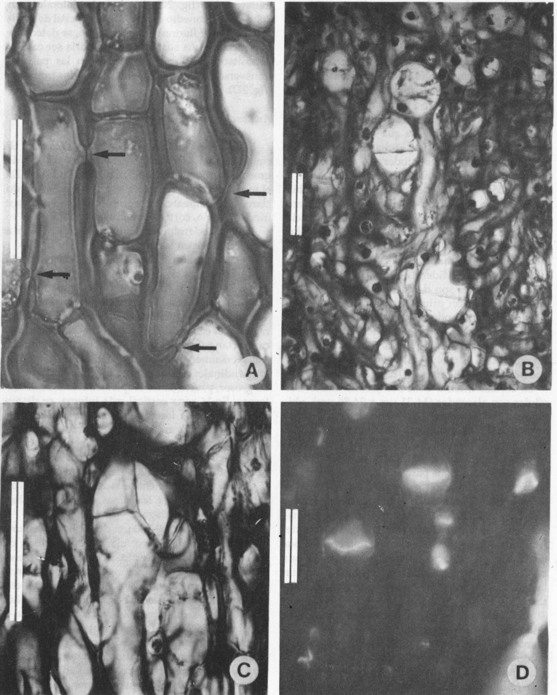
Fig. 2.-- Cortes longitudinales de rama. A: Células de la corteza interna, mostrando campos de puntuación primarios (flechas). B: Médula, mostrando filamentos trompeta y filamentos menores. C: Médula, mostrando una conexión entre 3 células trompeta a nivel de sus paredes transversales. D: Microfotografía de fluorescencia, mostrando la ubicación de la posible calosa en los filamentos trompeta medulares. Escalas: 50 \mu m.
