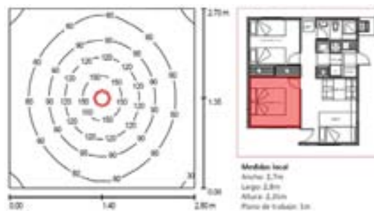
Figura 4: Ejemplo de análisis de la iluminación artificial, en lux, en el plano de trabajo (1m de altura).
