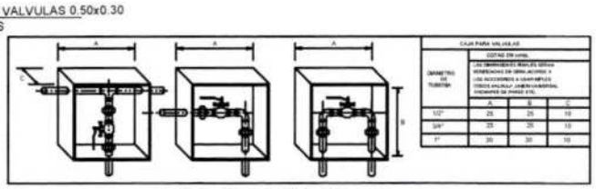
CAJA PARA VALVULAS
