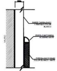
DETALLE N° 03 UNION PARED CERAMICA
