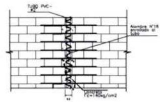
DETALLE DE TUBERIA DE VENTILACION ELEVACION ESC. 1/20
