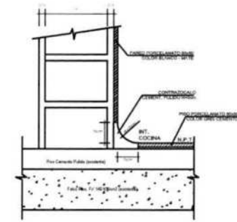
DETALLE N° 01-A CONTRAZOCALO SANITARIO INT. COCINA * DETALLE A UTILIZAR EN UNION PISO (CERAMICA) Y PARED (CERAMICA)
