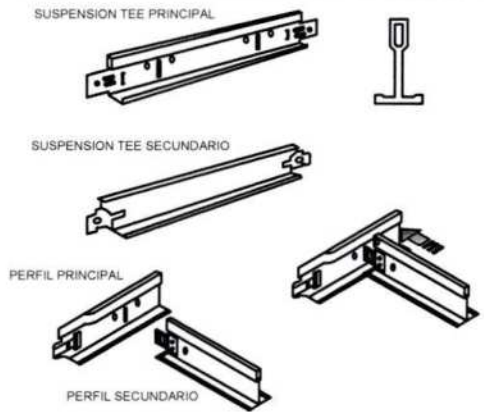
UNION ENTRE PERFILES DE AUTO-ENSAMBLE
