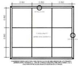
DETALLE N° 01 REVESTIMIENTO PORCELANATO EN PISO
