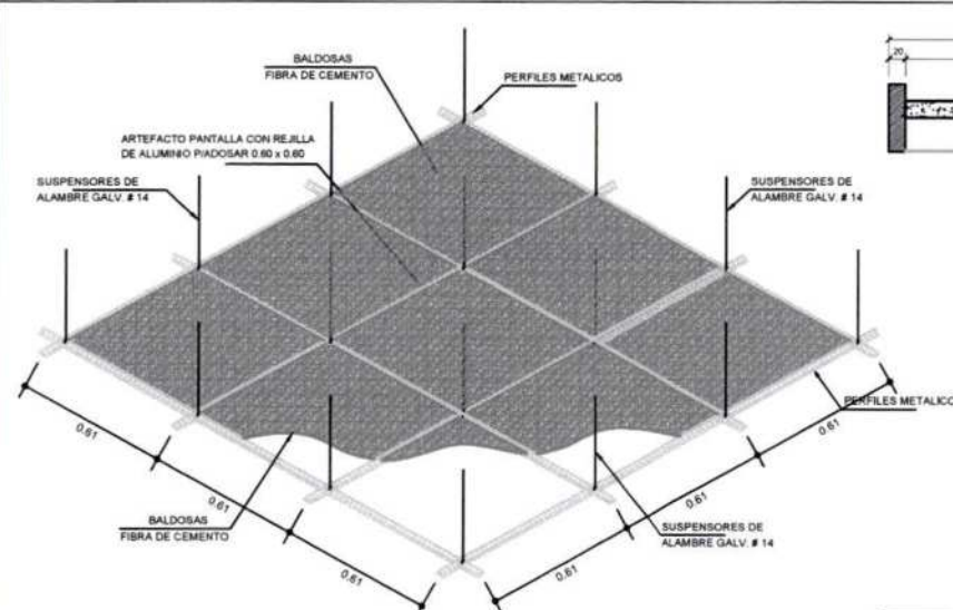
Vista Superior Cielorrasos Suspendedos
