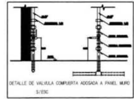
DETALLE DE VALVULA COMPUERTA ADOSSADA A PANEL MERO S/ENC
