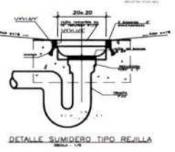
DETALLE SUMIDERO TIPO REJILLA ESC. 1/8
