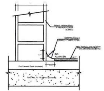
DETALLE N° 01-B CONTRAZOCALO SANITARIO INT. ALMACEN * DETALLE A UTILIZAR EN UNION PISO (CERAMICA) Y PARED (TARRAJEADO)
