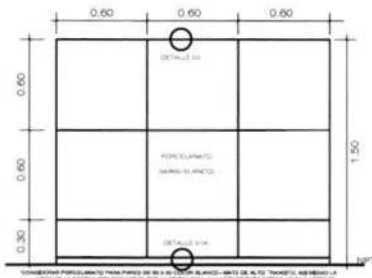
DETALLE N° 02 REVESTIMIENTO PORCELANATO EN PARED
