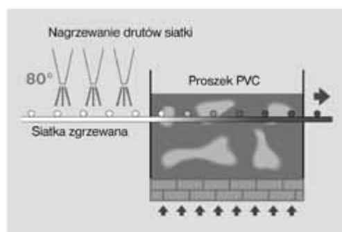
Fluidyzacja (sintercoating)
