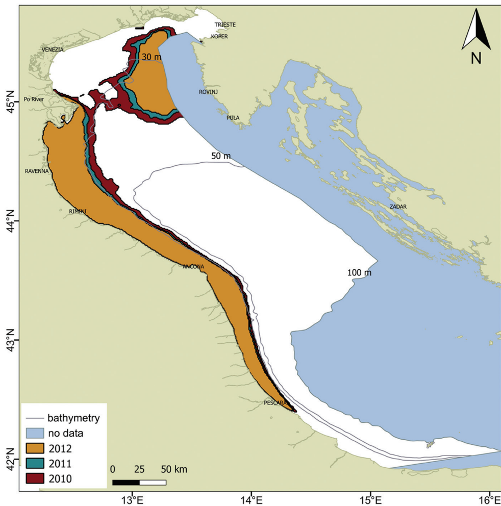
Fig. 5: A. kagoshimensis hotspot map: 2010 to 2012.
