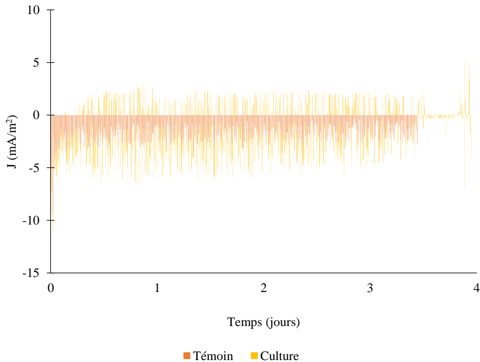
Figure 4.15 : Chronoampérogrammes sur une électrode en plaque d'acier polarisée à -0,3 V/ECS.
