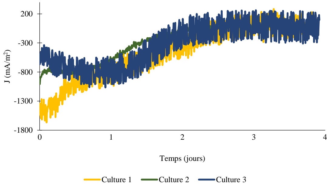
Figure 4.17 : Chronoampérogrammes enregistrés à un potentiel (vs ECS) = -0,3V avec une électrode en feutre de carbone.
