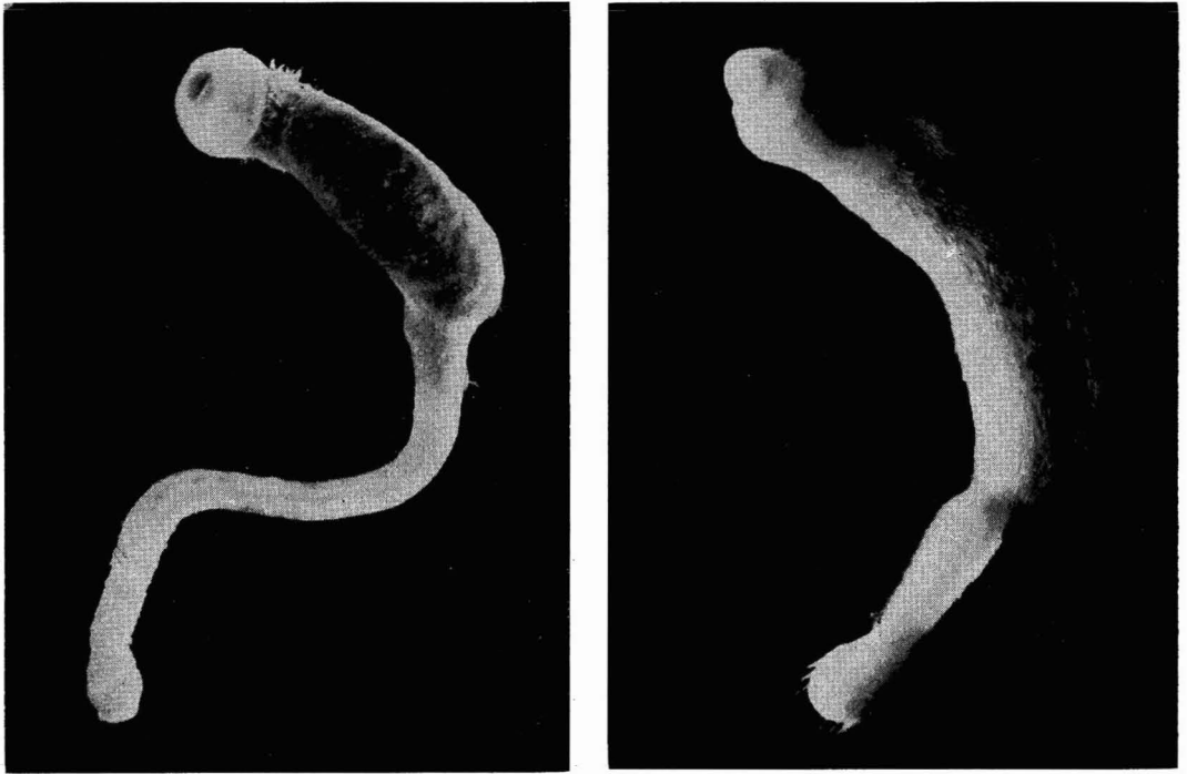
FIG. 12. Crystallophrisson bartmani . Left, Sta. 2302-53. Right, Sta. 2644-54.
