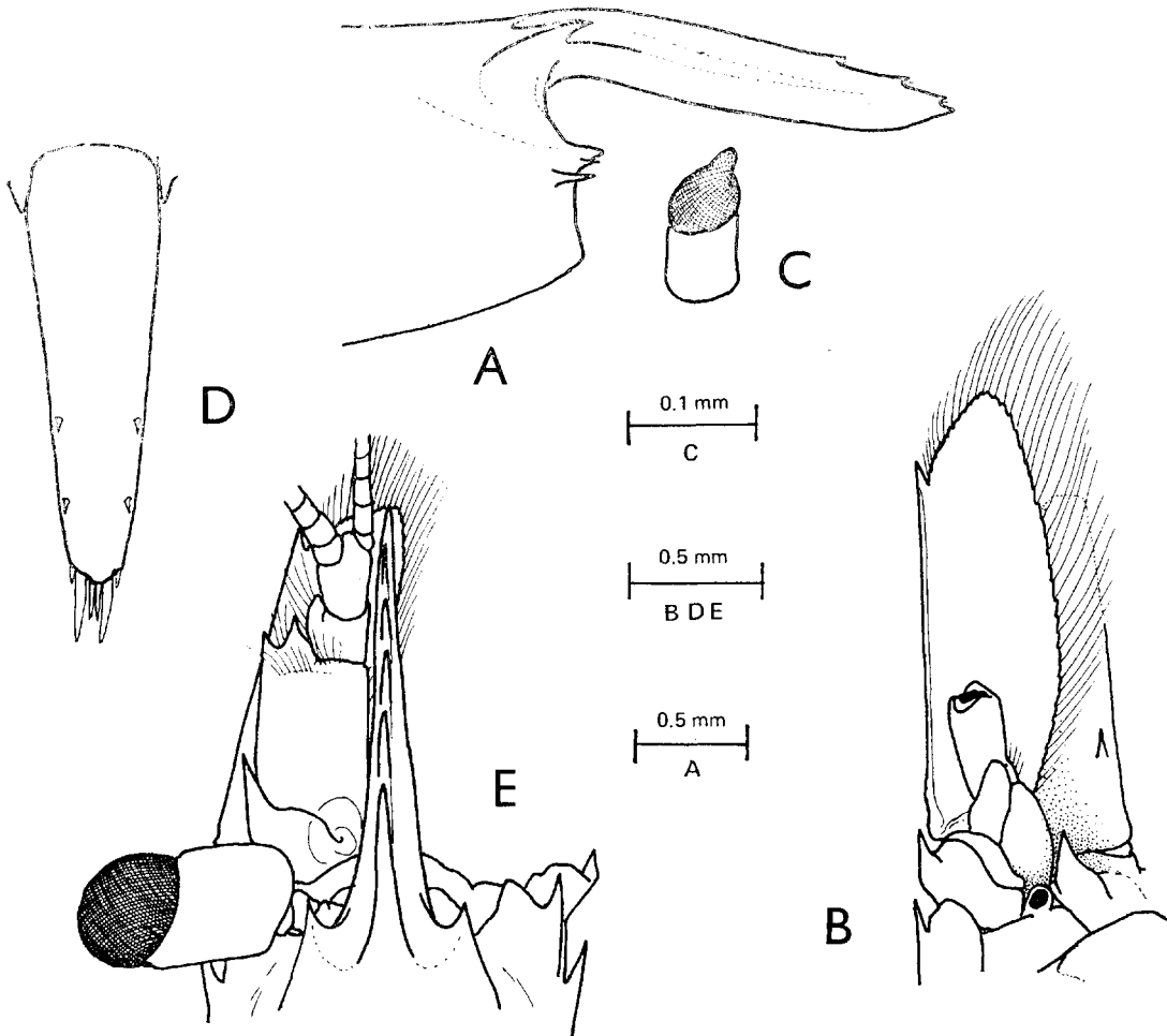
FIG. 4. — Periclimenes ceratophthalmus Borradaile : A, anterior carapace and rostrum ; B, epistomal region ; C, eye ; D, telson. — Periclimenes commensalis Borradaile : E, anterior carapace, rostrum and antennae. (A-D, ♂ ; E, ovigerous ♀.)
