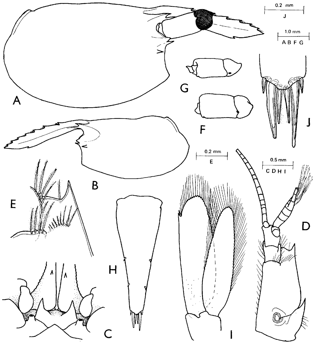
FIG. 1. — Periclimenes amboinensis (De Mau) : A, B, anterior carapace and rostrum ; C, epistomal region ; D, antennule ; E, idem , distolateral angle of proximal segment ; F, G, eyes ; H, telson ; I, uropod ; J, posterior telson spines. (A, F, ovigerous ♀ ; B-E, G-J, ♂.)
