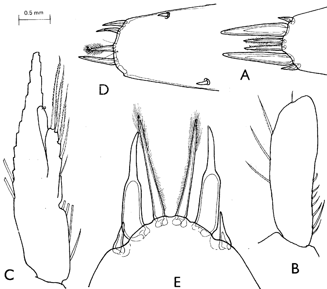
FIG. 6. — Periclimenes ceratophthalmus Borradaile ♂ : A, posterior telson spines ; B, endopod of first pleopod ; C, endopod of second pleopod. — Araiopontonia odorhyncha Fujino & Miyake, ♂ : D, posterior telson spines. — Paranchistus nobilii Holthuis, ovigerous ♀ : E, posterior telson spines.
