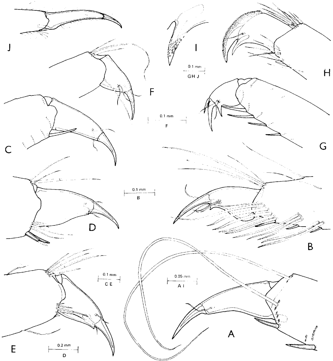
FIG. 7. — Dactyls of third pereiopods : A, Periclimenes affinis (Zehntner) ; B, Periclimenes amboinensis (De Man) ; C, Periclimenes amygone De Man ; D, E, Periclimenes brevicarpalis (Schenkel) ; F, Periclimenes ceratophthalmus Borradaile ; G, Araiopontonia odontorhyncha Fujino & Miyake ; H, Paranchistus serenei sp. nov. ; I, idem , accessory tooth ; J, Pycnodonta hyotis Hipeau-Jacquotte. (A, C, G, propodal setae largely omitted ; B, F, G, ♂ ; D, E, ovigerous ♀.)
