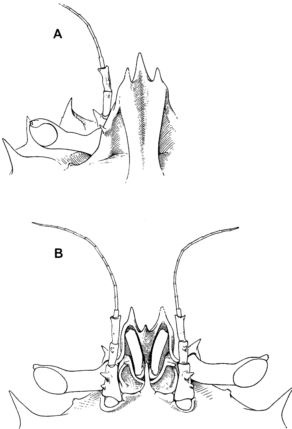
FIG. 1. — Cyrtomaia ericina sp. nov., holotype, ♂ 18 × 22 mm, côte sud de la Nouvelle-Calédonie, 220-390 m, INGRES coll. (MP-B7240) : région fronto-orbitaire (× 7), vue dorsale (A) et vue ventrale (B). (Pilosité non représentée.)
