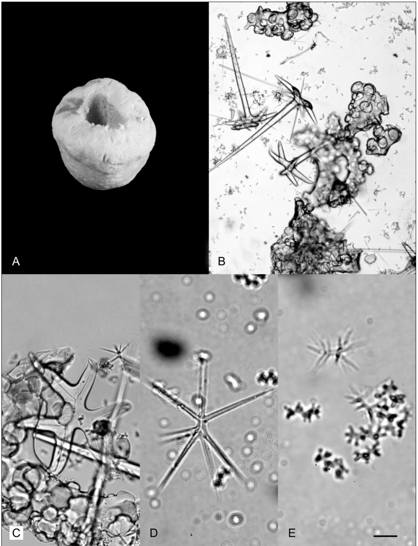
Figure 10. Neoschrammeniella antarctica n. sp.
