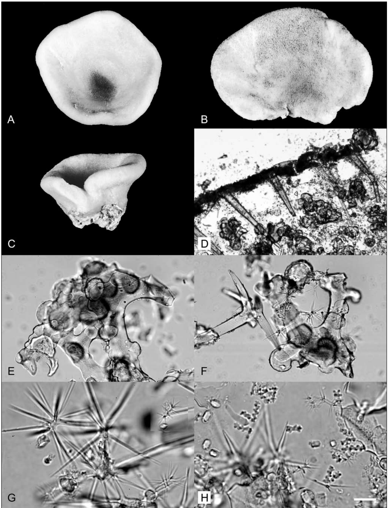
Figure 9. Neoschrammeniella fulvodesmus (Lévi & Lévi, 1983).
