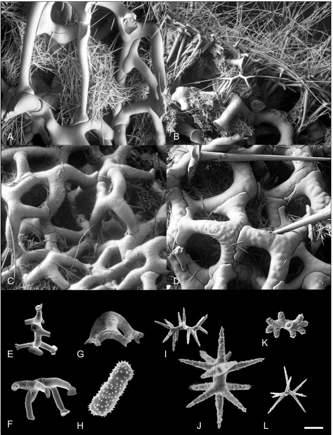
Figure 22. A, E, I, K, Pleroma turbinatum Sollas, 1888; B, C, F, H, L, P. menoui Lévi & Lévi, 1983; D, G, J, P. aotea Kelly, 2003.
