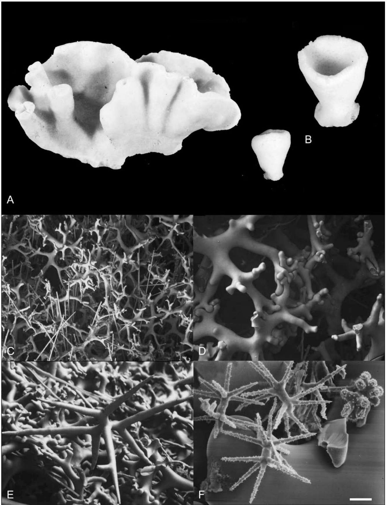
Figure 8. Reidispongia coerulea Lévi & Lévi, 1988.
