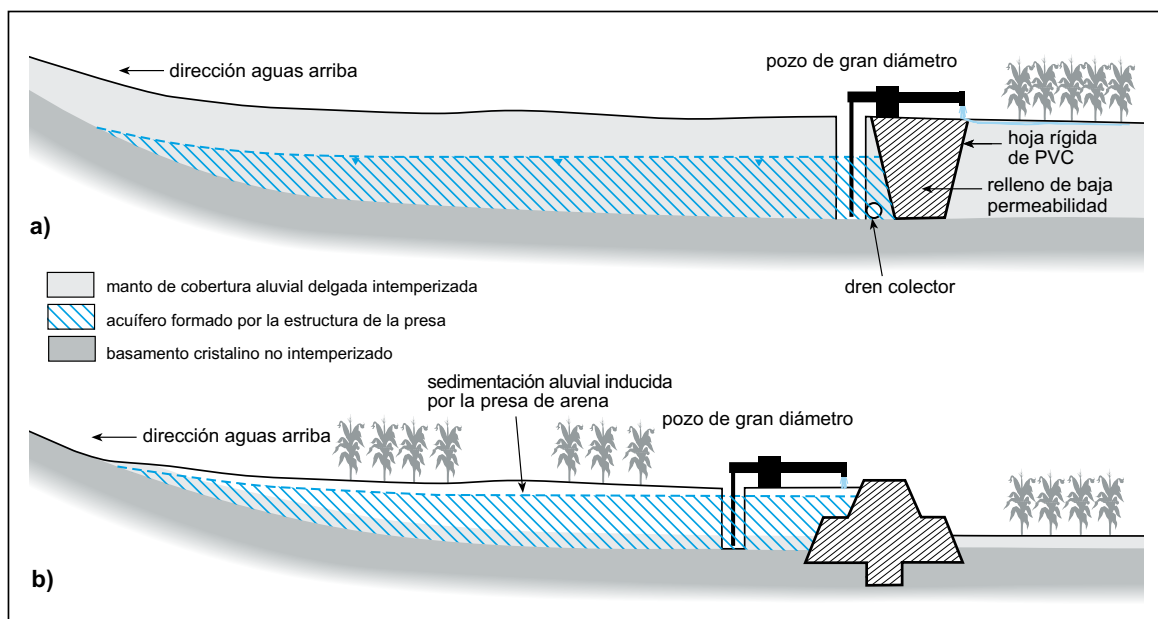
Figura 3: Secciones longitudinales esquemáticas para ilustrar (a) presas de agua subterránea y (b) presas de arena
