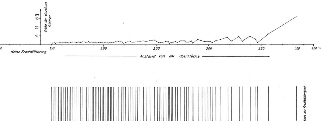
Abb. 4. Diagramm der Frostblätter in der Sandgrube von Haselbach aufgrund einer Vermessung.
