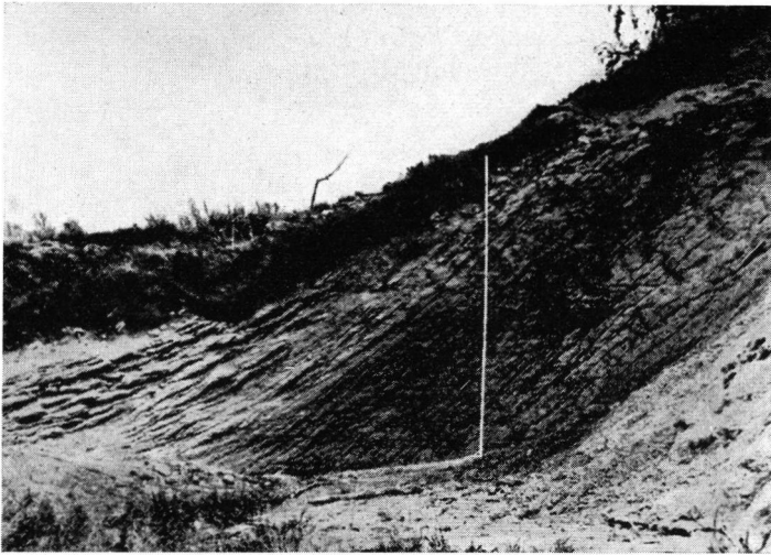
Abb. 3. Sandgrube bei Haselbach, Kreis Ellwangen. Horizontal geschichteter, zersetzter Stubensandstein mit eiszeitlicher Frostblättrung, die etwa parallel zum Hang verläuft.
