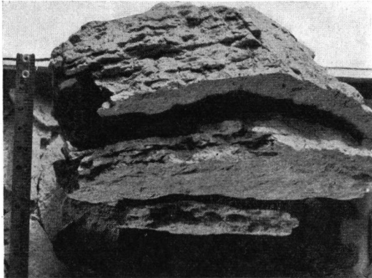
Abb. 2. Lößlehm aus der Lehmgrube Unterweißach, Kreis Backnang mit Frostblätterstruktur vom Winter 1953/54. Die Probe ist aus der alten Baggerwand entnommen. Die Blätter liegen parallel zur Baggerwand.
