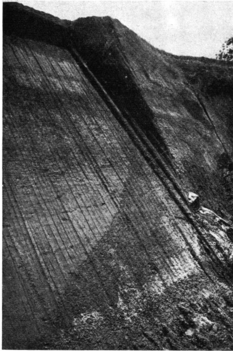
Abb. 1. Lehmgrube Unterweißach, Kreis Backnang. Die Grubenwand ist etwa 6 m hoch. Rechts die alte Baggerfront von 1954, links die neue von 1955. Der Frost ist im Winter 1953/54 ca. 60 cm tief senkrecht zur alten Baggerwand eingedrungen. Die Aufblätterungszone ist vom Bagger 1955 unter spitzem Winkel angeschnitten worden. Die Frostgrenze ist in der neuen Baggerwand deutlich zu erkennen, sie verläuft von der linken unteren Ecke zur Mitte des Bildes. Die fossile Frostblättrigkeit in horizontaler Richtung ist ebenfalls erkenntlich. Man beachte, daß nach unten die Blätter immer dicker werden.
